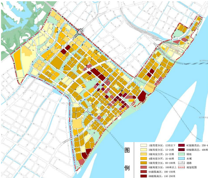
高度控制图
