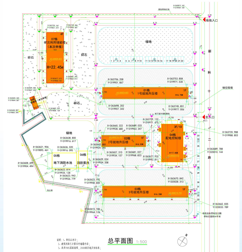
更改后 cad 总平面图
