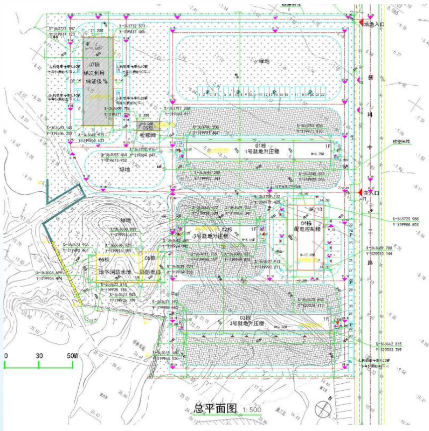
原方案 cad 总平面图
