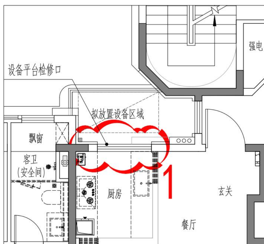
4#5#6#7#住宅 二~二十四层局部平面图（变更后）
