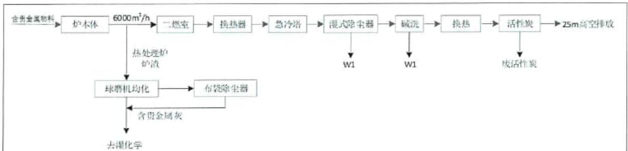
热处理工艺流程及产污环节图
