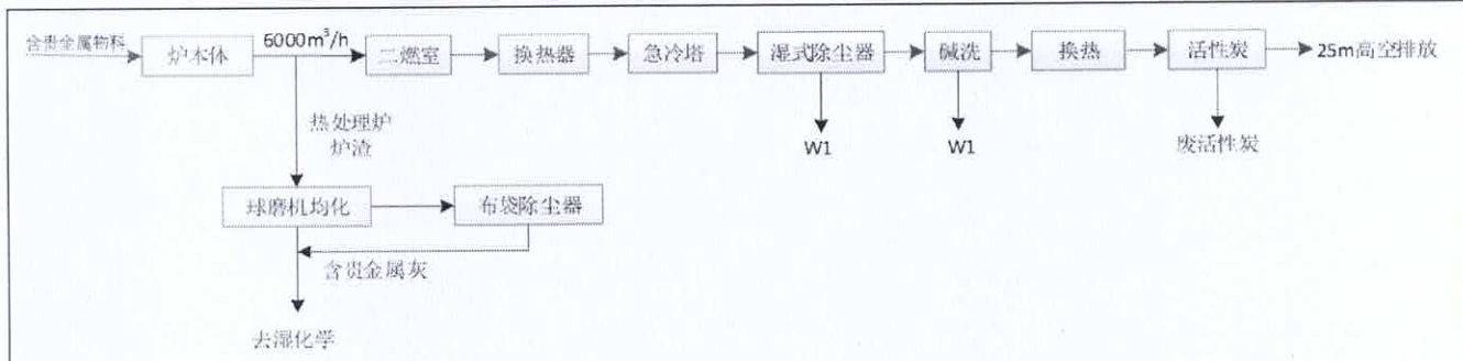
热处理工艺流程及产污环节图
