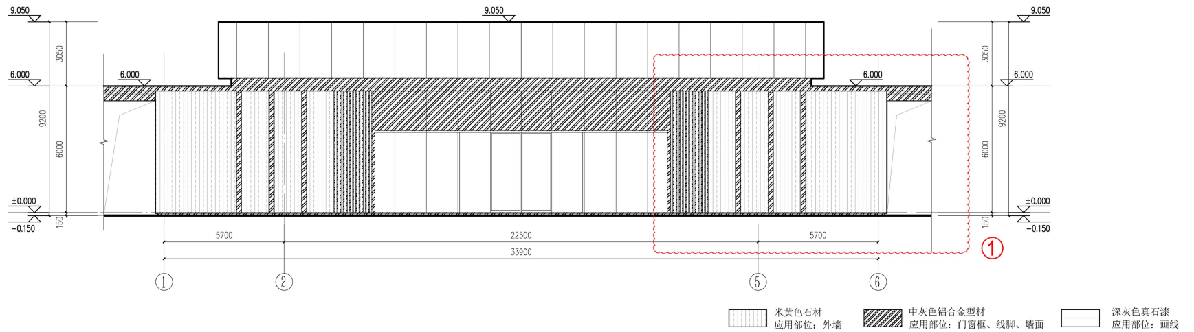
7#楼 1~6轴立面图变更前
