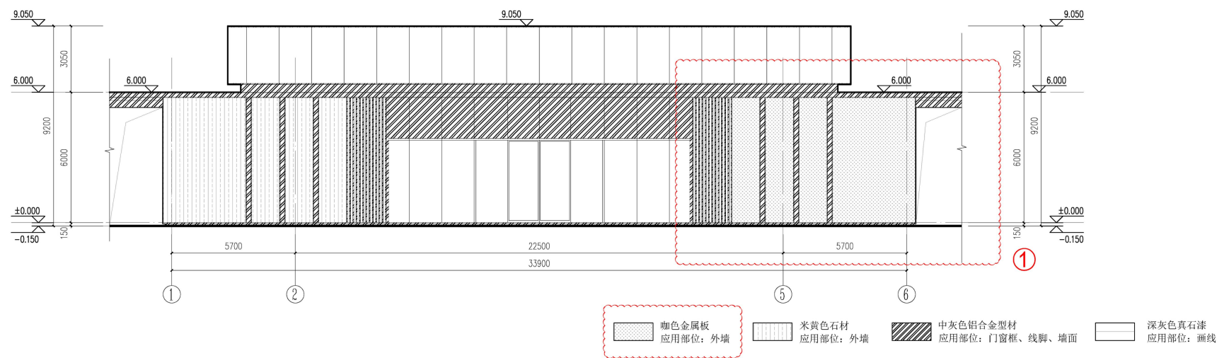
7#楼 1~6轴立面图变更后
