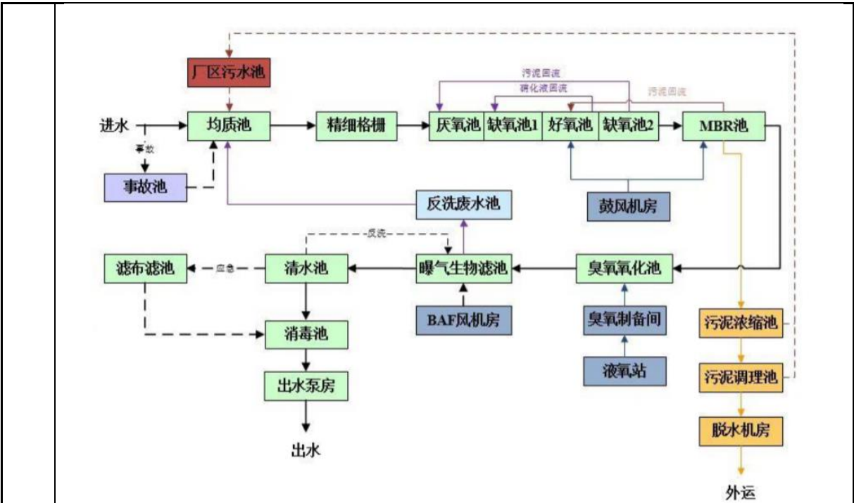
图 4-1 改造后污水处理厂二期工程污水处理流程图
