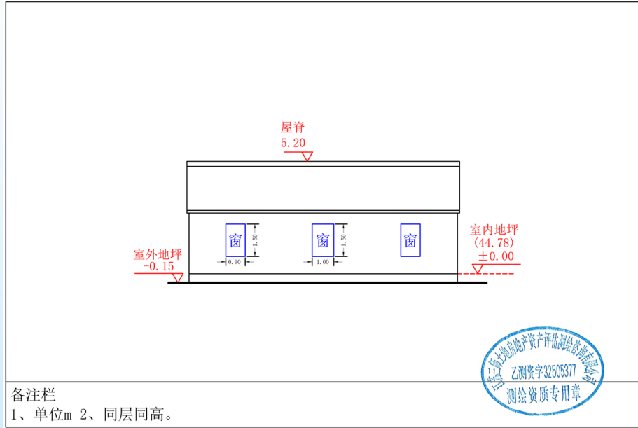
大厂街道王山头组80号北立面
