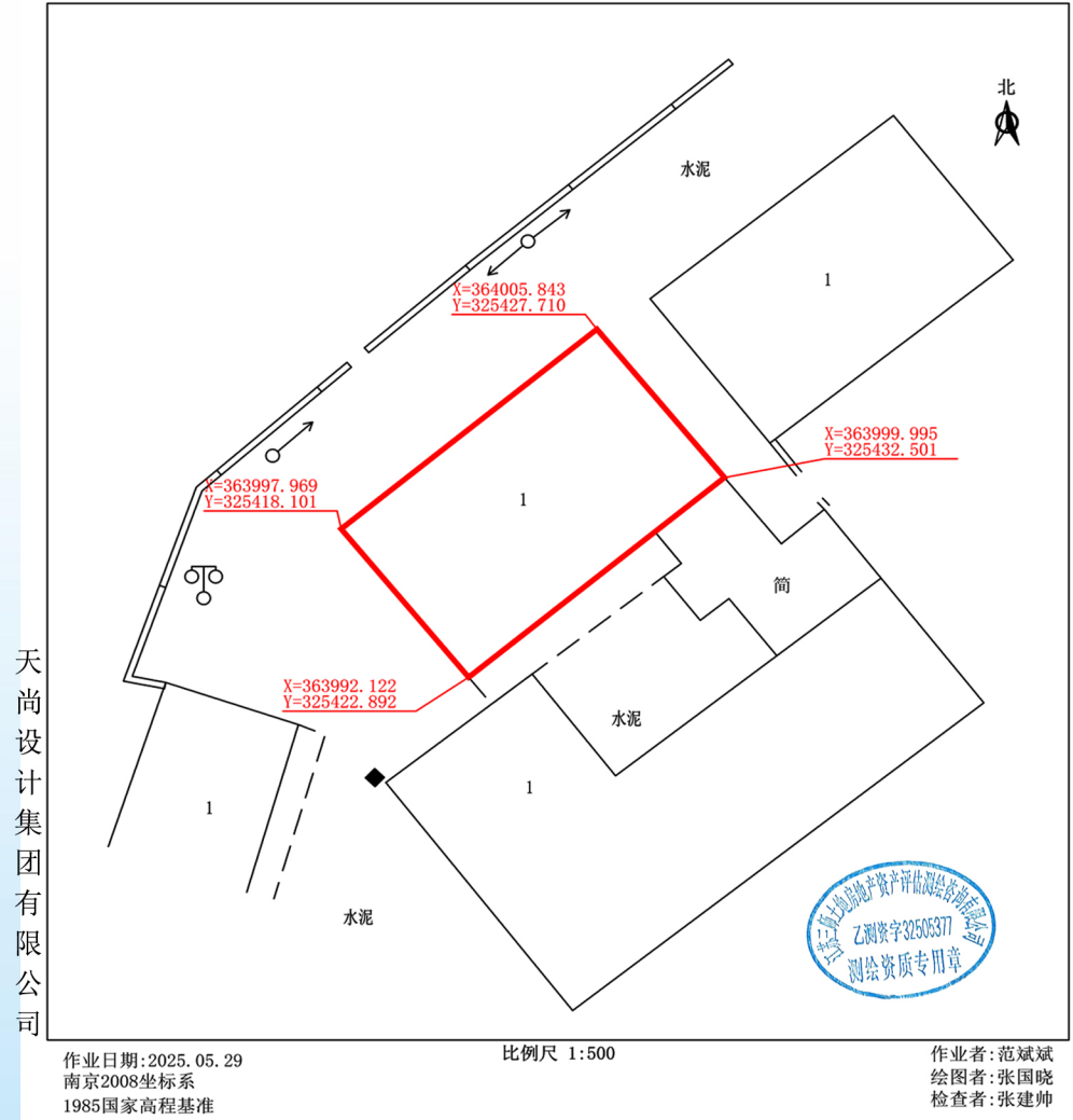
大厂街道王山头组80号平面图
