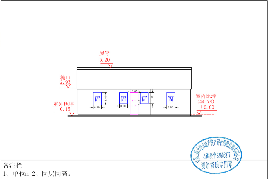
大厂街道王山头组80号南立面
