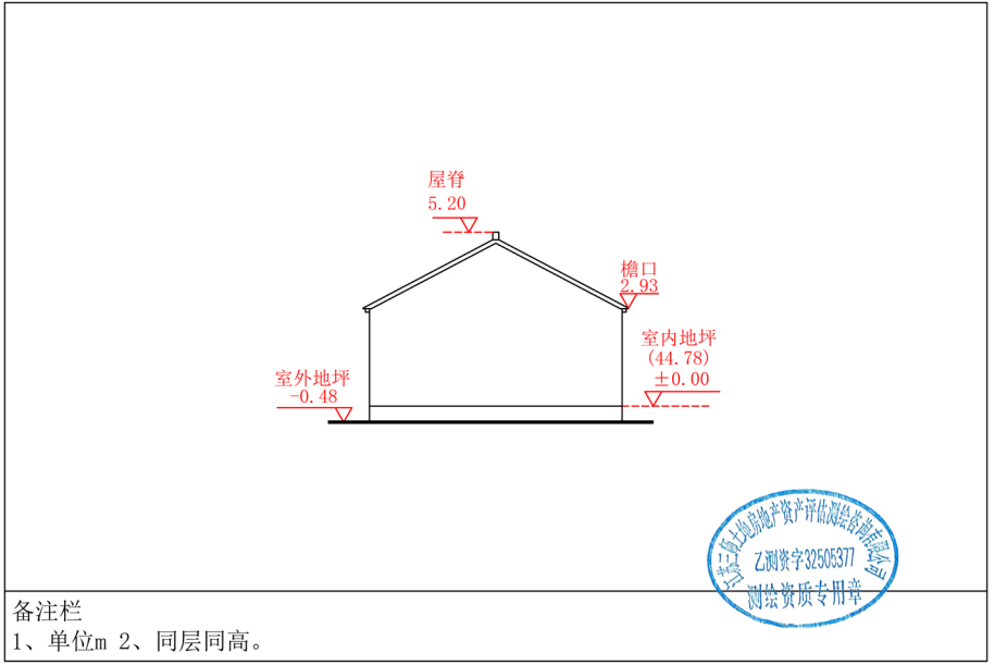
大厂街道王山头组80号东立面
