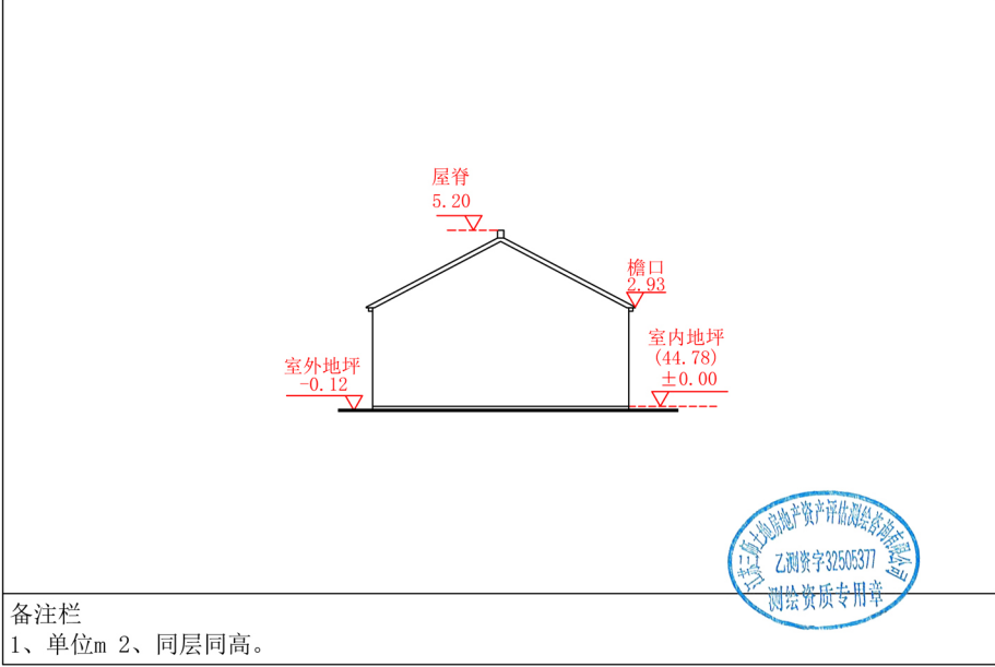
大厂街道王山头组80号西立面
