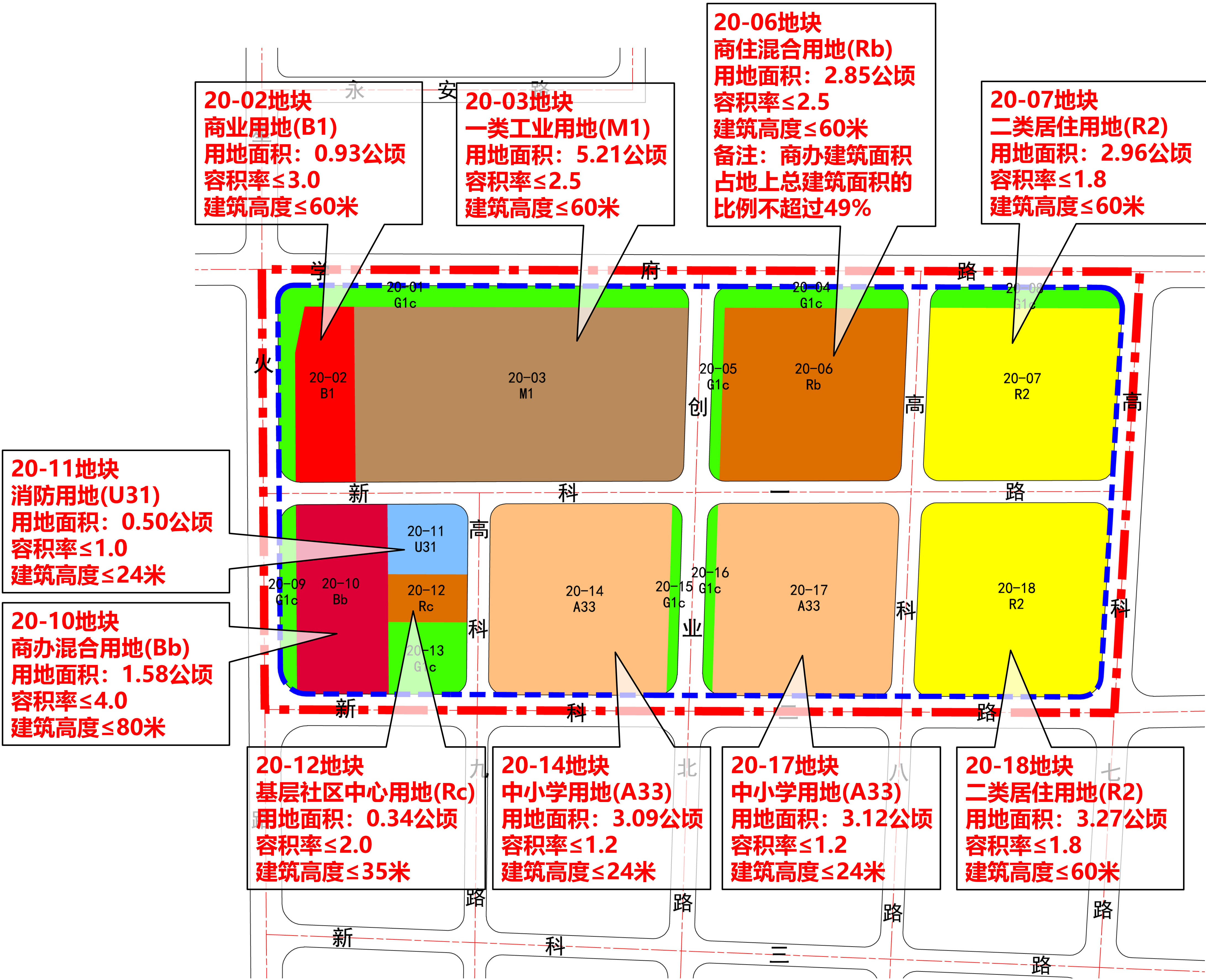
NJJBb040—20规划管理单元修改后图则
