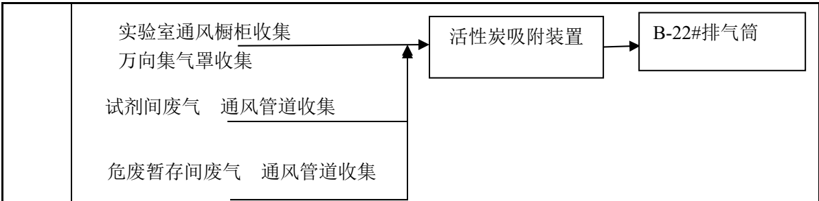
图 4-1 废气收集处理系统示意图
