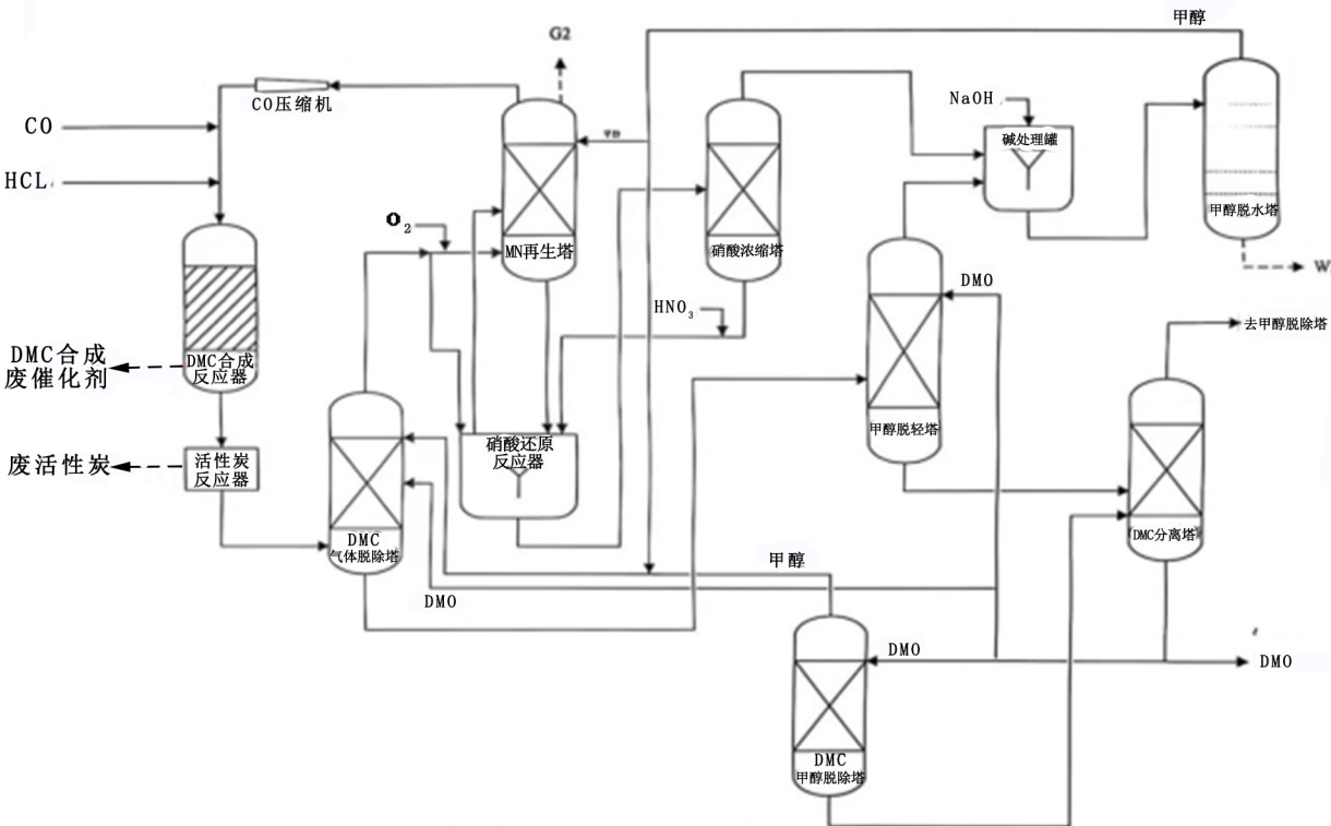
DMC 合成工艺流程及产污环节图
