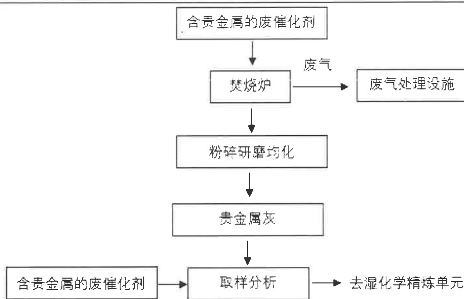
热处理单元流程图
