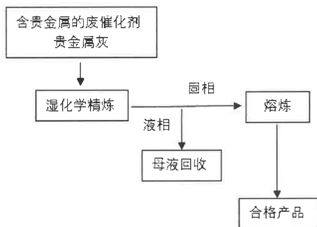
湿化学精炼单元流程图
