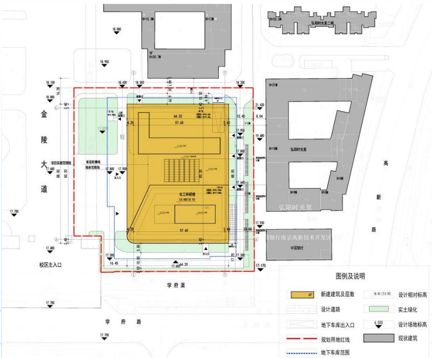
化工科研楼总平面
