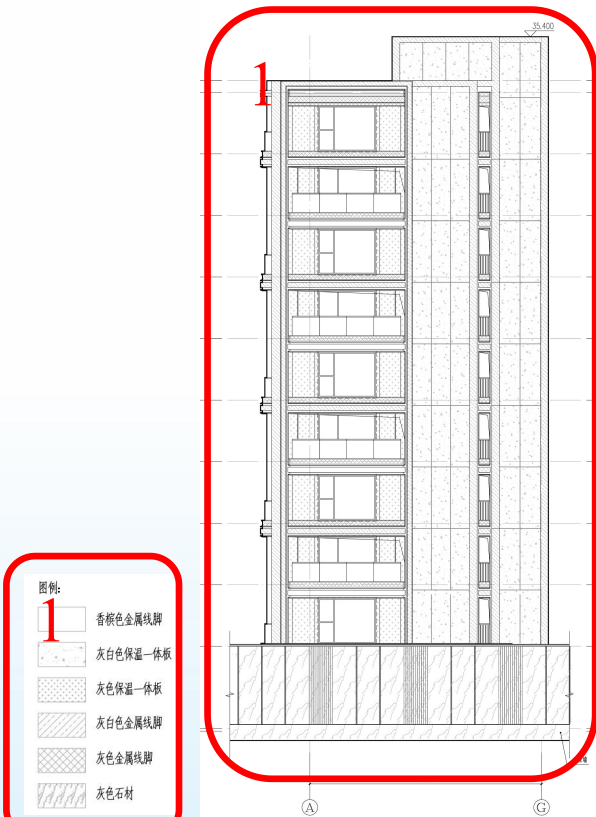
5#8# G-A 轴立面图
