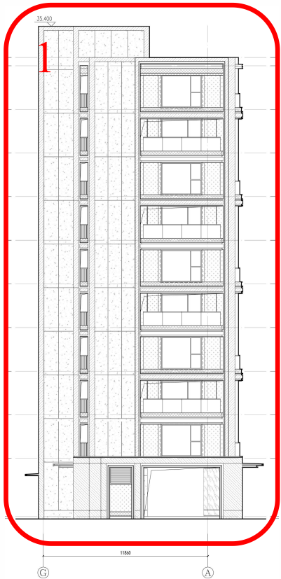
5#8# G-A 轴立面图
