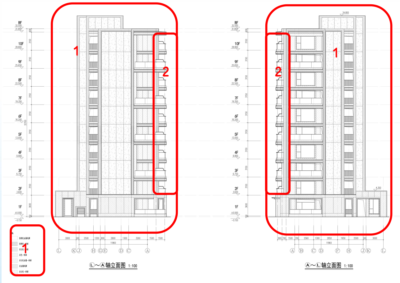
3# L-A 轴立面图
