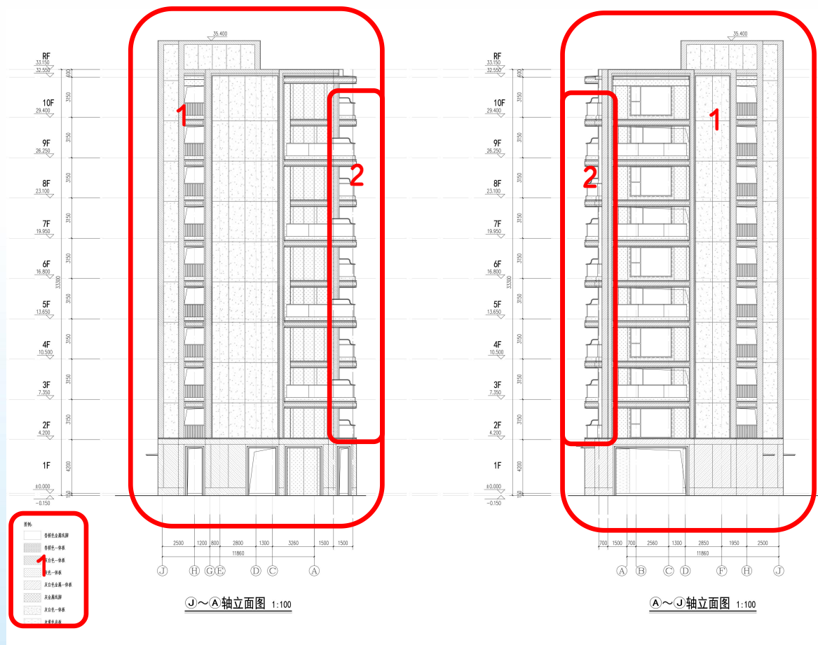
6#9# J-A 轴立面图
