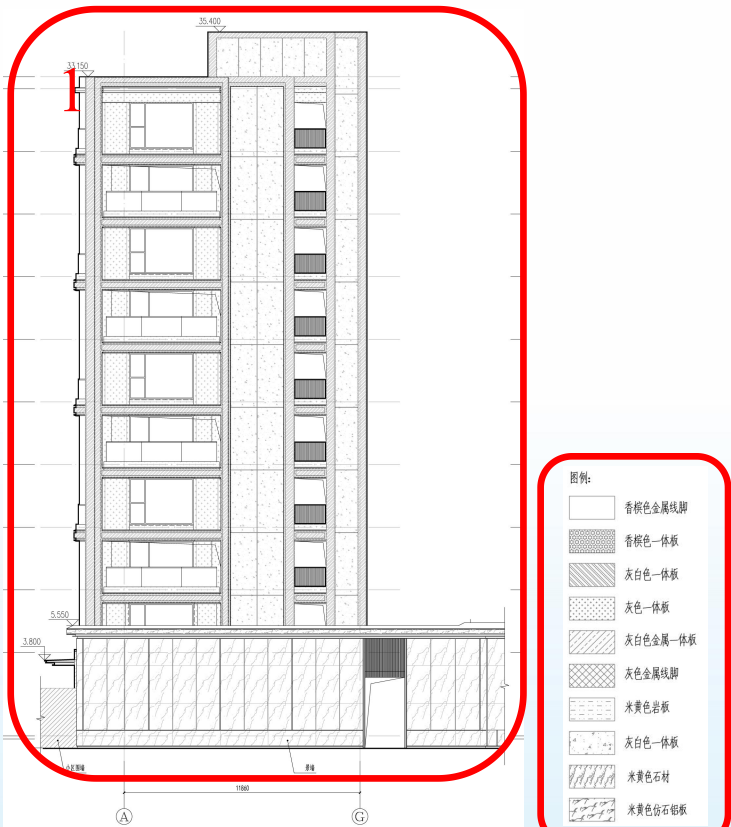
5#8# A-G 轴立面图
