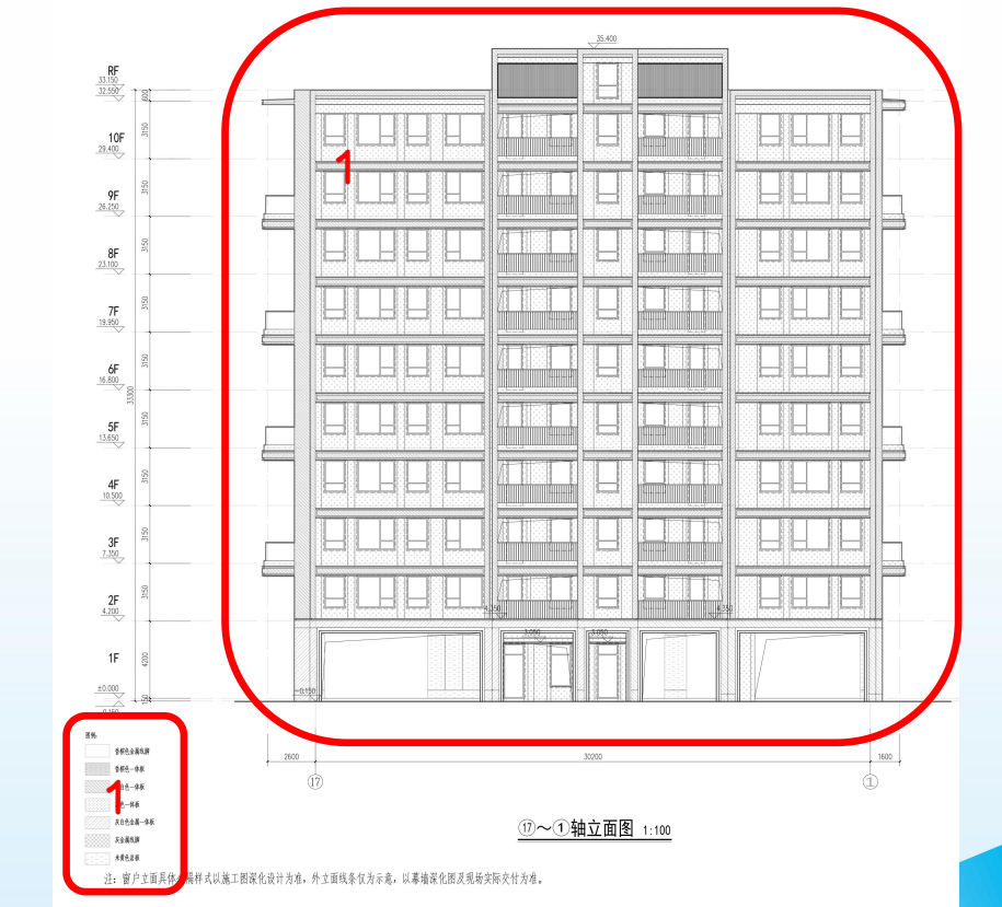
6#9# 17-1 轴立面图
