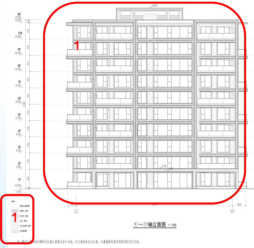
3# 1-17 轴立面图
