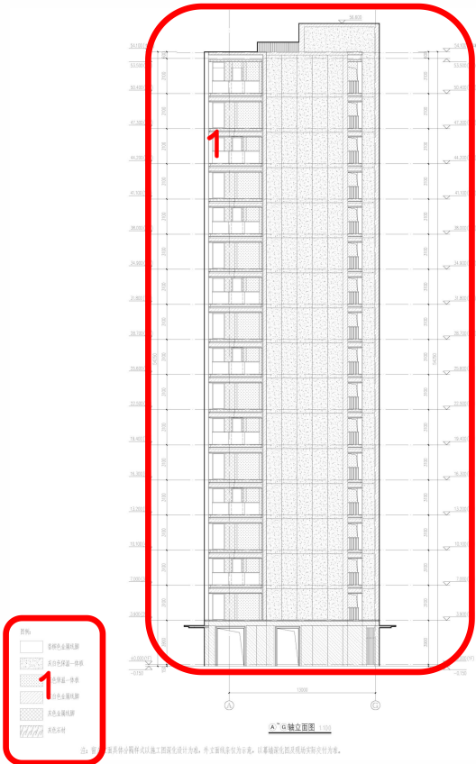
11# A-G 轴立面图
