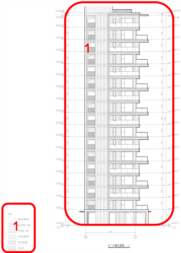
10# A-K 轴立面图
