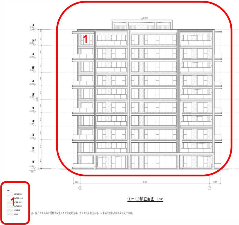
3# 1-17 轴立面图
