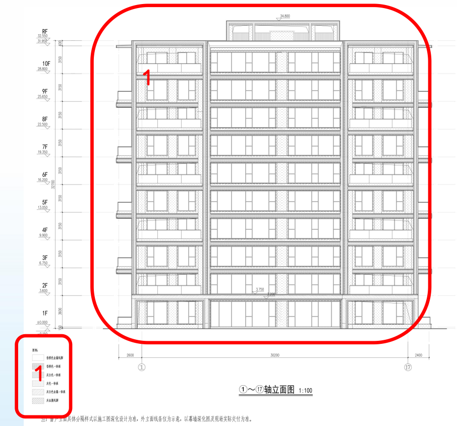
4# 1-17 轴立面图
