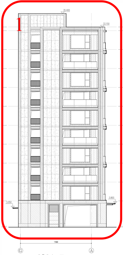
5#8# A-G 轴立面图
