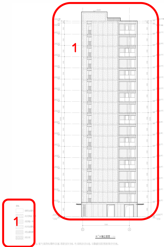
11# G-A 轴立面图
