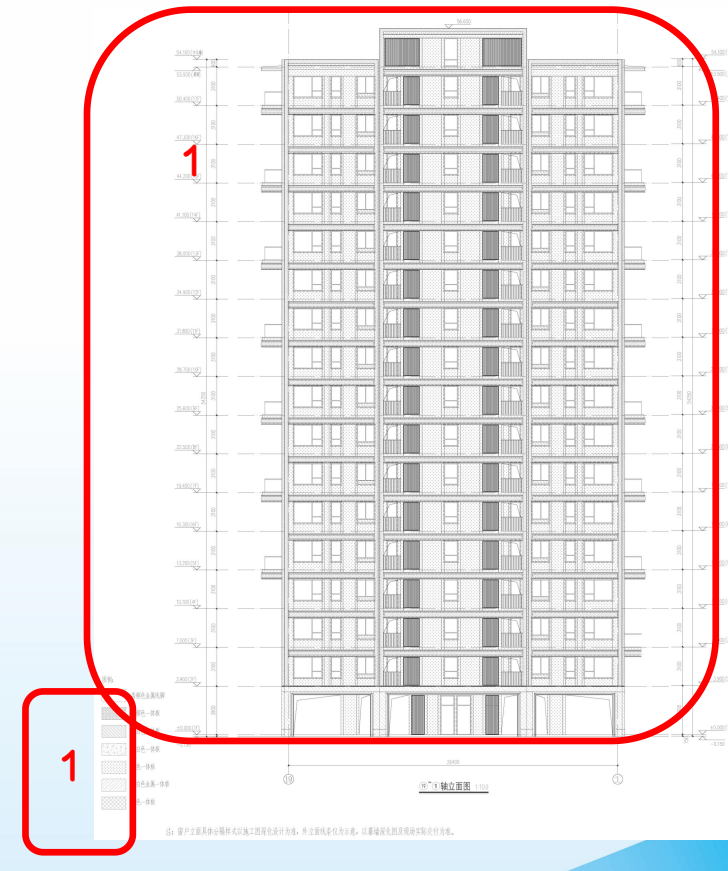
10# 19-1 轴立面图
