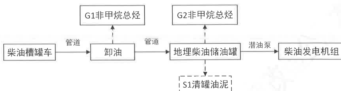
图 2-2 项目运行期工艺流程示意图
