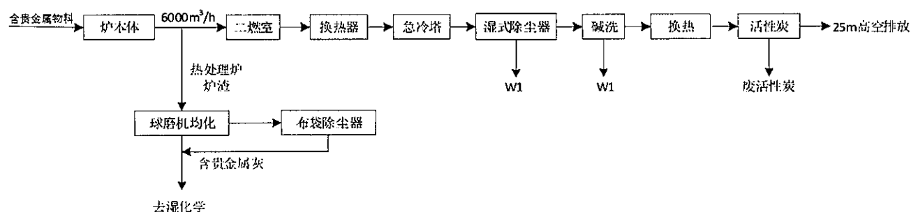
热处理工艺流程及产污环节图
