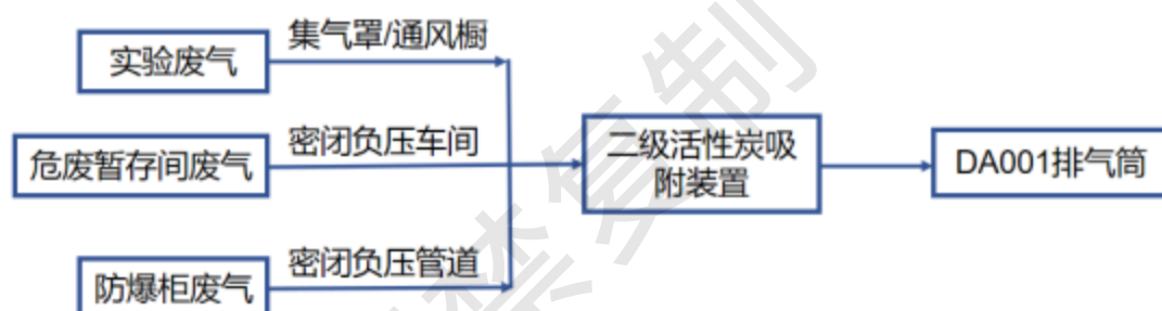
图 4-1 本项目废气收集治理示意图
