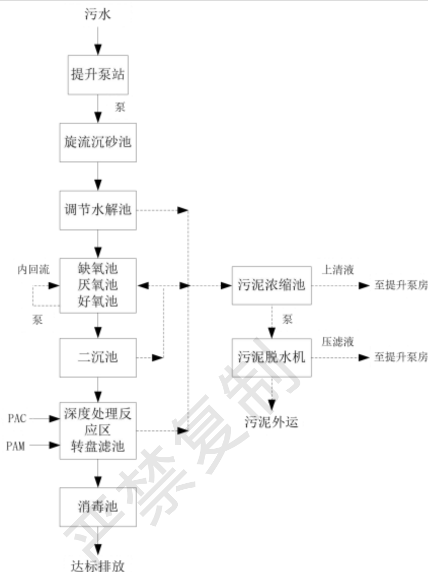
图 4-3 盘城污水处理厂处理工艺流程示意图
