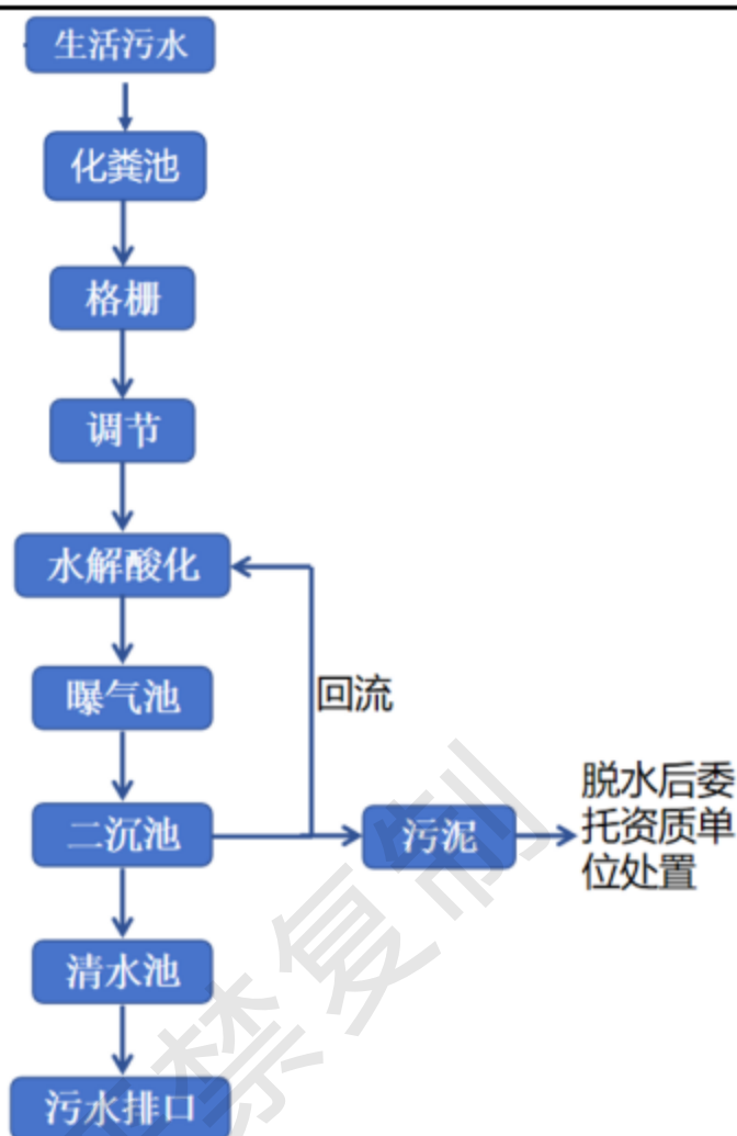
图 4-2 中丹园二期污水处理站工艺流程示意图
