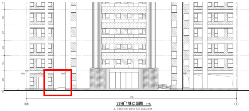
2#楼变更前 33 轴~1 轴局部立面图
