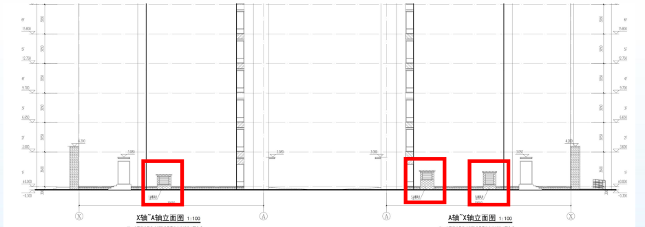
1#、5#楼变更后局部侧立面图
