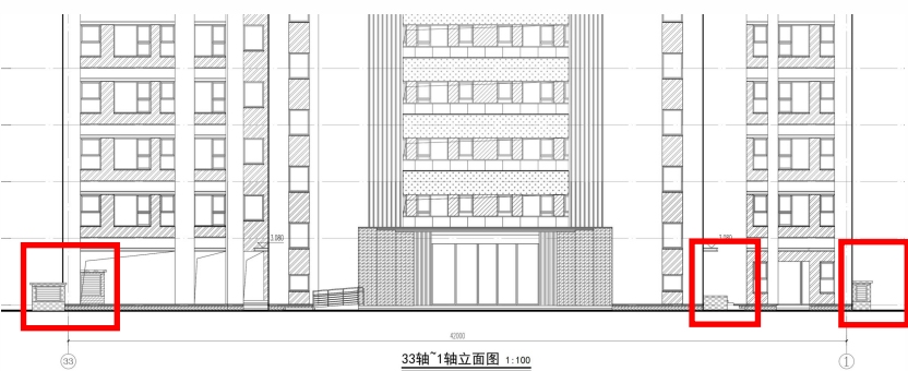
4#楼 33~1 轴变更后局部立面图
