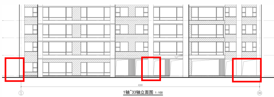
4#楼 1~33 轴变更前局部立面图
