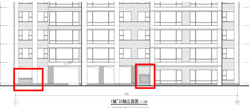
2#楼变更后 1 轴~33 轴局部立面图
