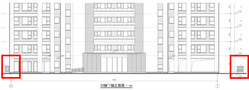
3#楼变更后 33 轴~1 轴局部立面图
