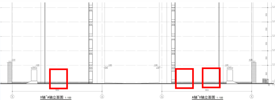
1#、5#楼变更前局部侧立面图
