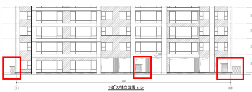
4#楼 1~33 轴变更后局部立面图
