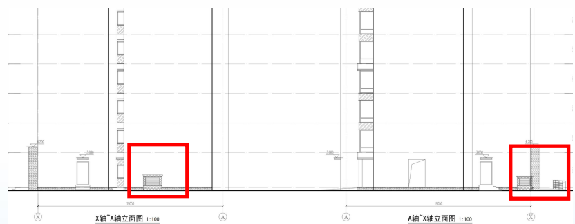
4#楼变更后局部侧立面图
