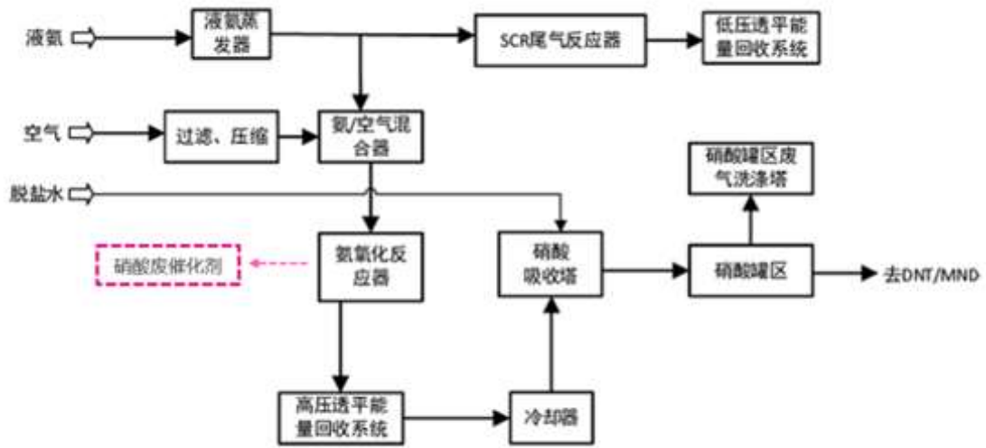
硝酸生产工艺流程图
