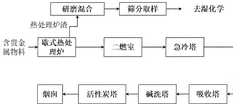
热处理工艺流程及产污环节图
