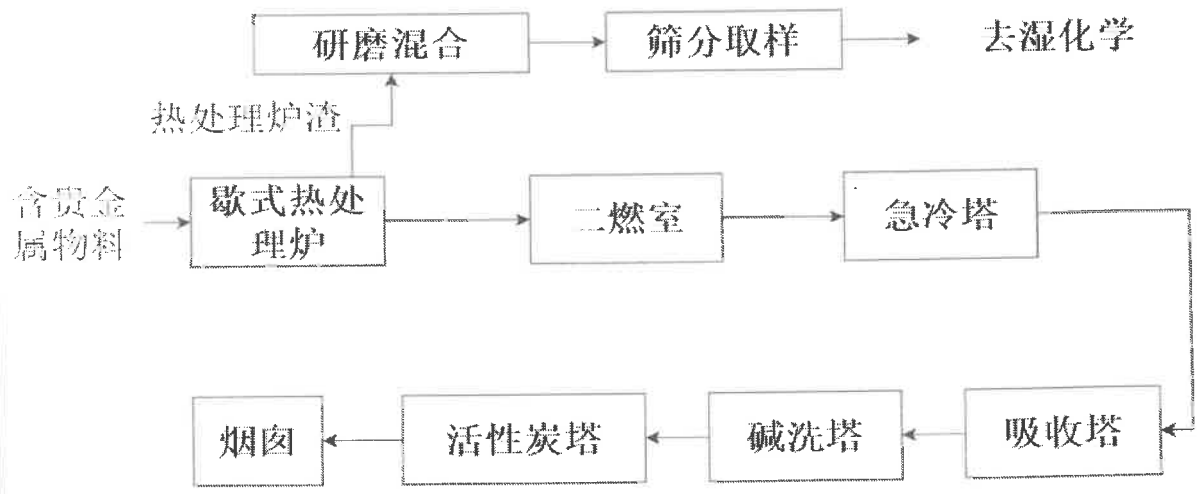
热处理工艺流程及产污环节图
