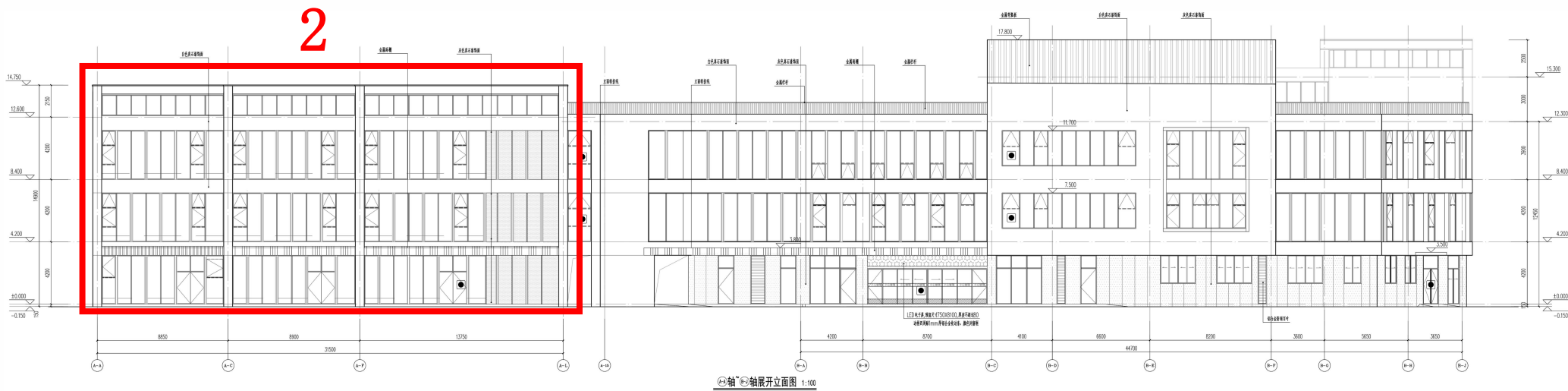
变更前（A-A 轴~B-J 轴展开立面图）
