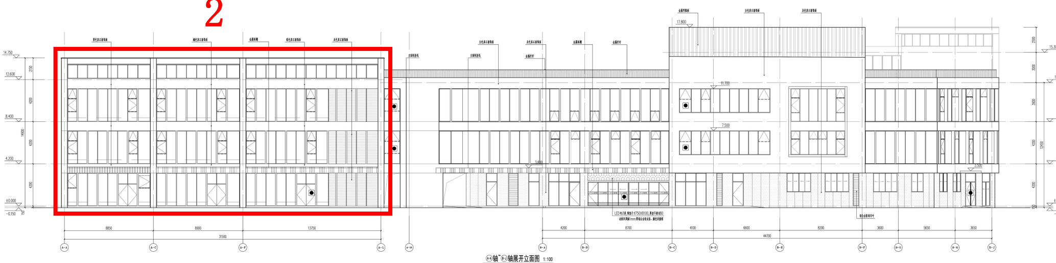
变更后（A-A 轴~B-J 轴展开立面图）
