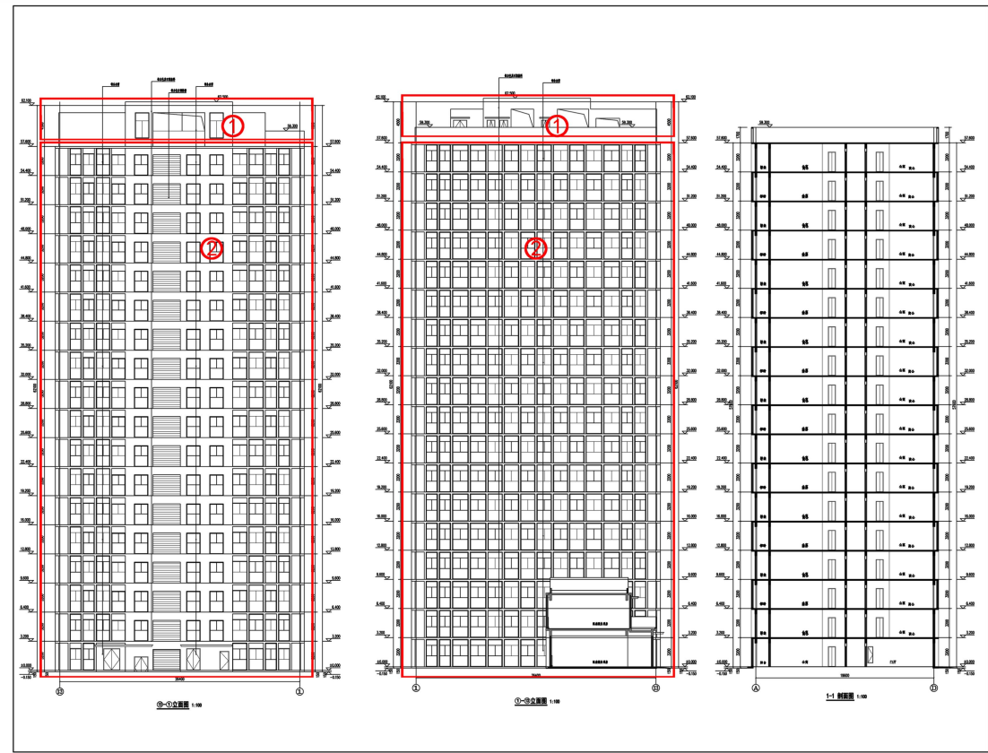
04#楼 1~13、13~1 轴立面变更后
