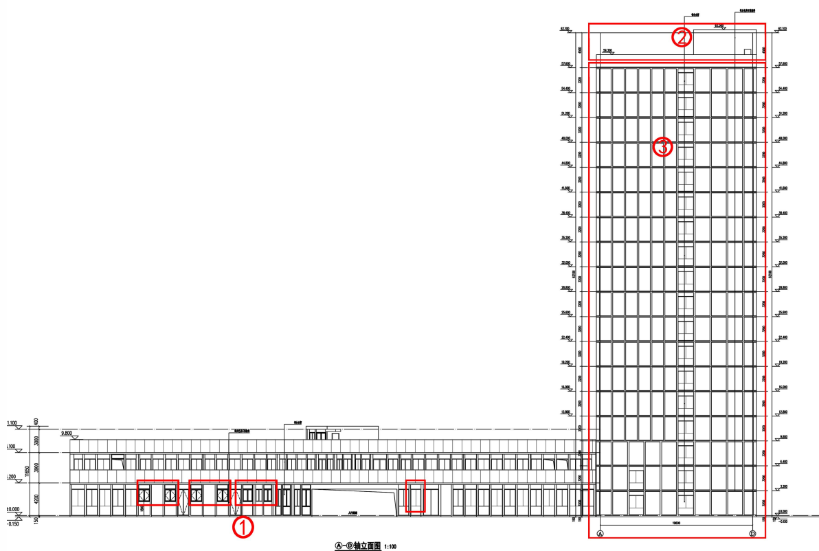
04#楼裙房 A-D 轴立面变更后
