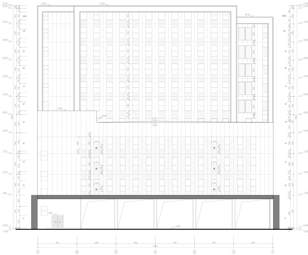
⑦轴~①轴立面图 1:100
