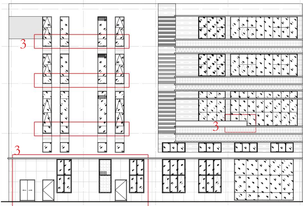
变更后 02 栋南、北立面图（09 栋为镜像布置）
