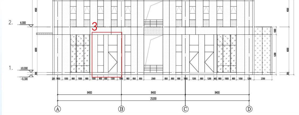
变更前 01 栋 1 轴 -7 轴立面图
