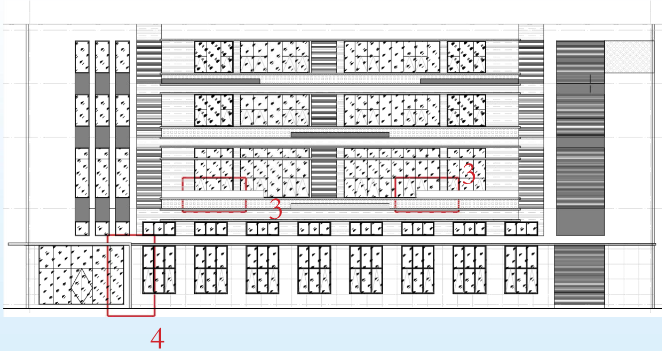
变更前 10 栋南、北立面图
