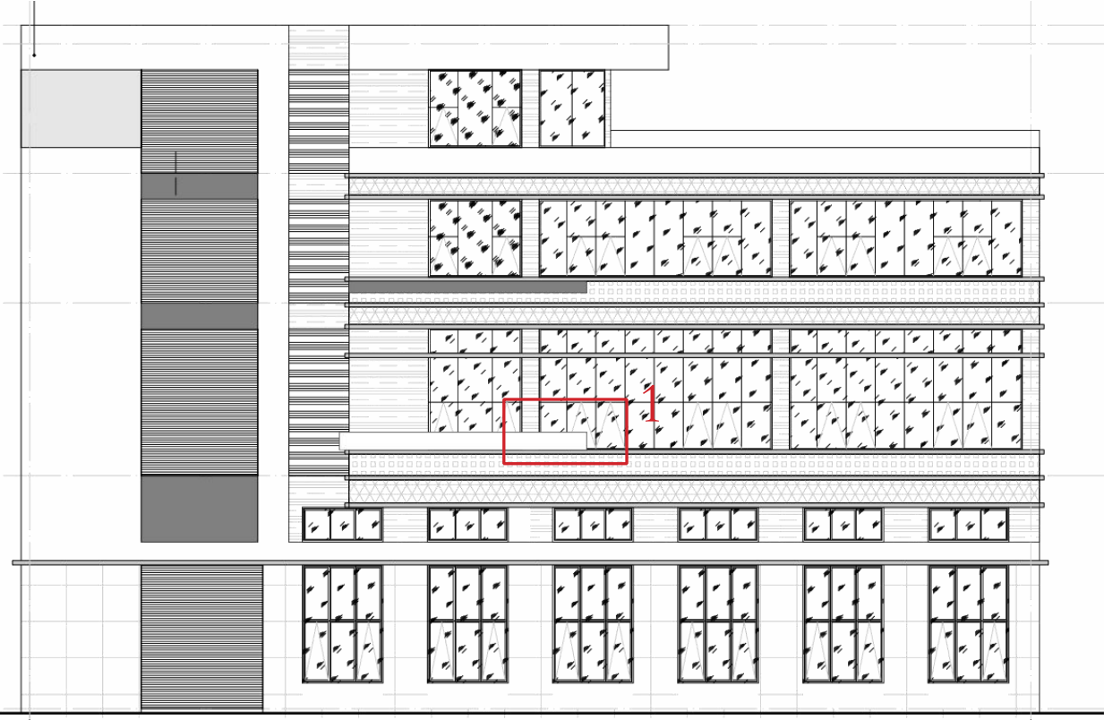
变更前 05 栋北立面图（06、07 栋为镜像布置）
