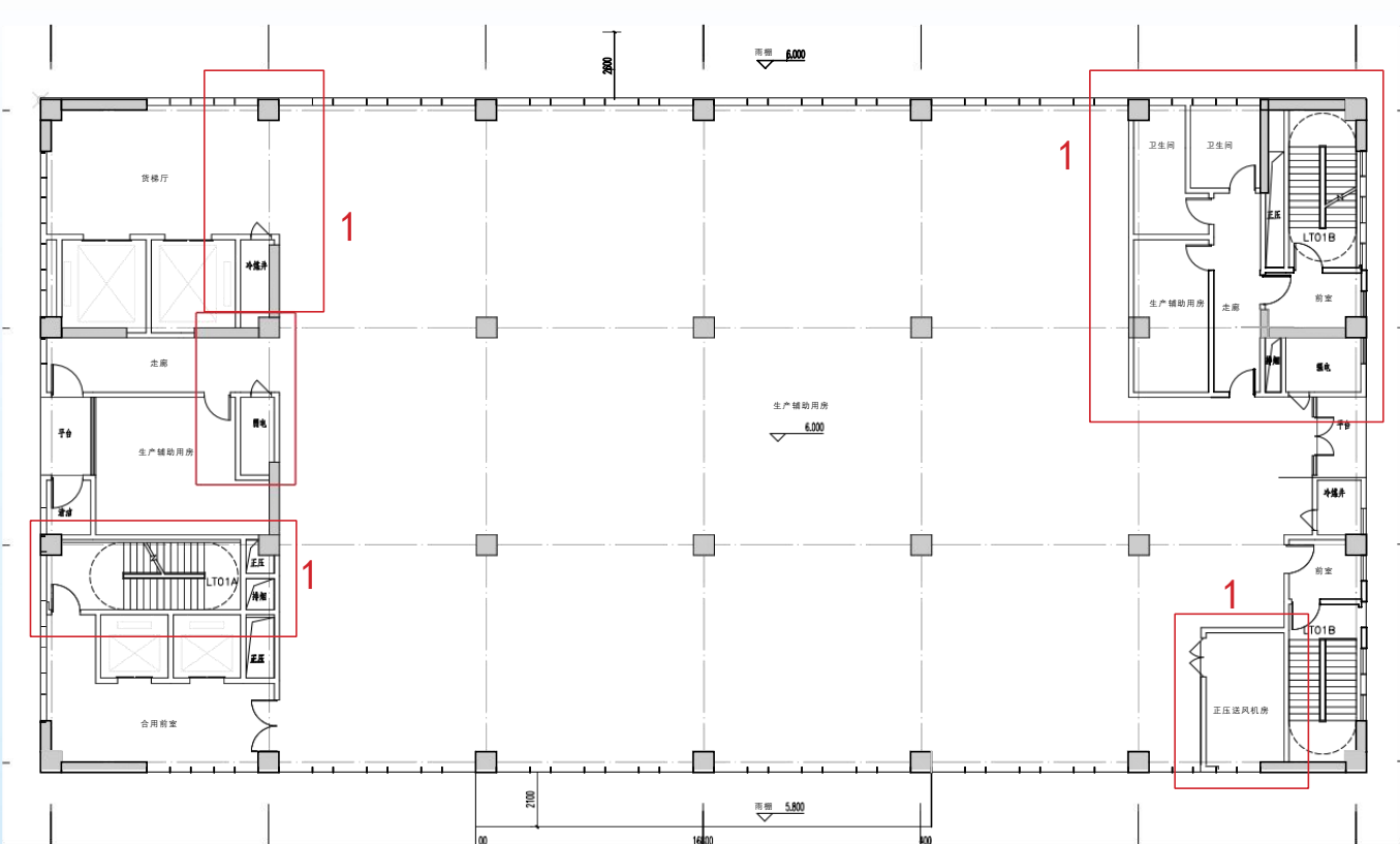
变更前 01 栋二层平面图
