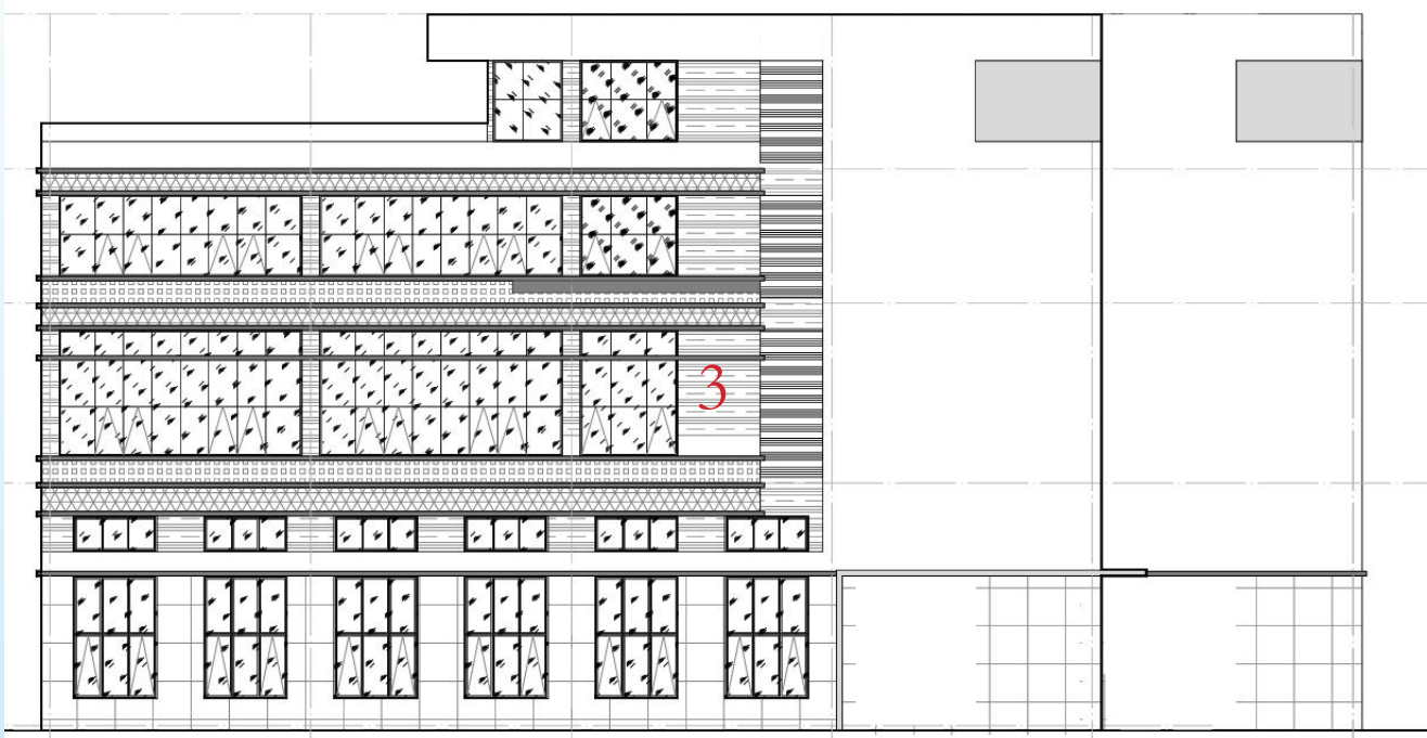
变更后 08 栋北立面图
