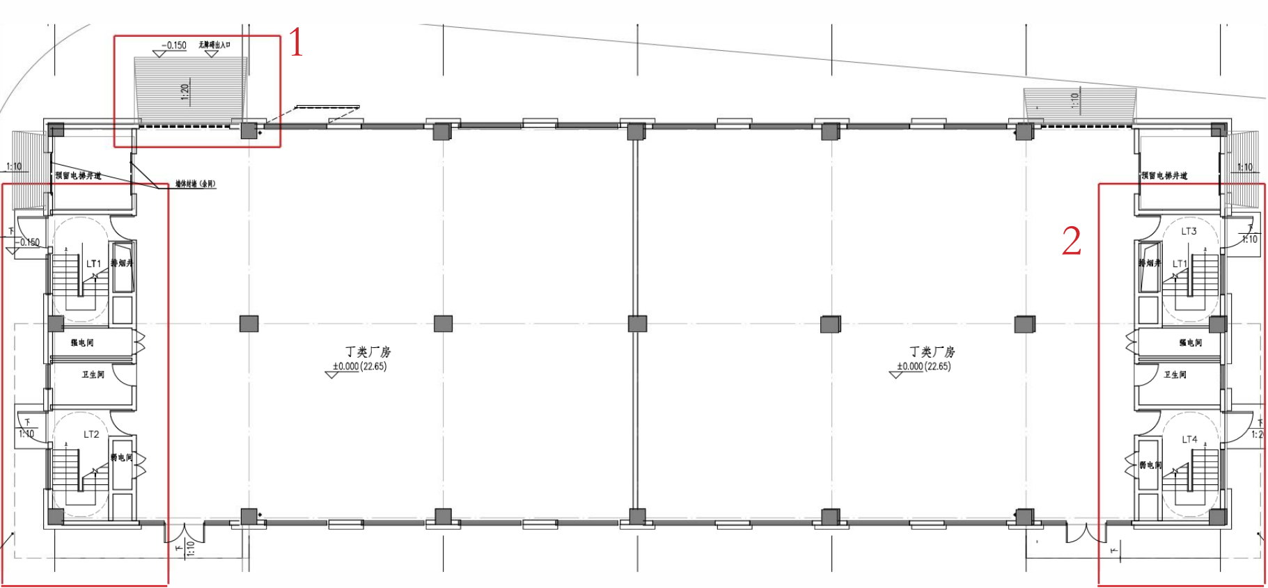
变更后 03 栋平面图
