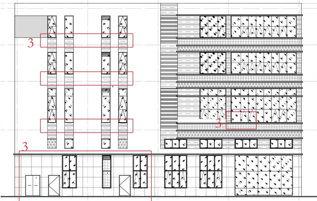
变更前 02 栋南、北立面图（09 栋为镜像布置）
