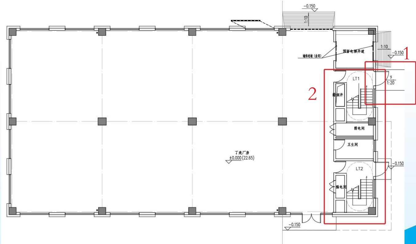
变更后 05 栋一层平面图 (06、07 栋为镜像布置)
