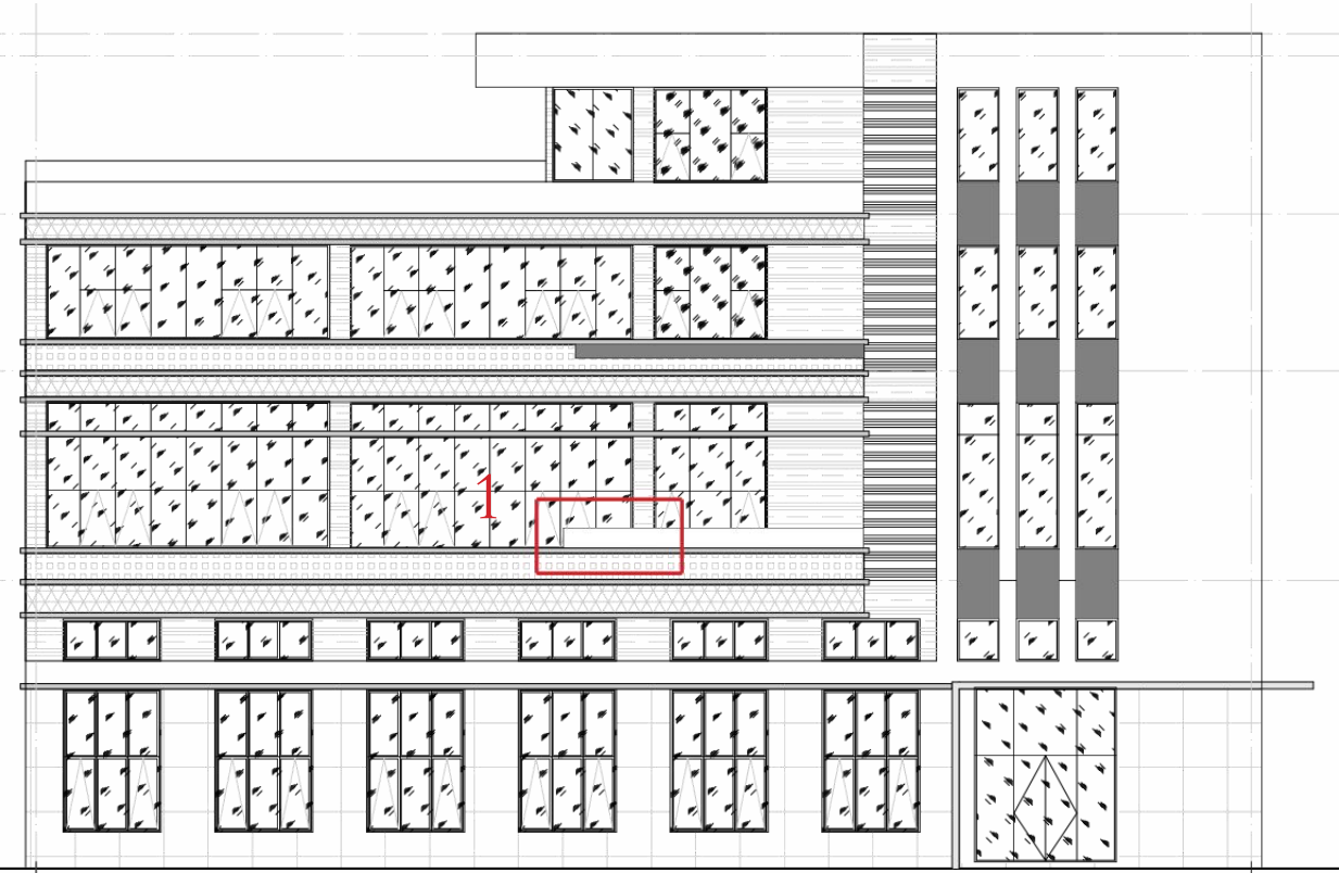
变更前 05 栋南立面图（06、07 栋为镜像布置）
