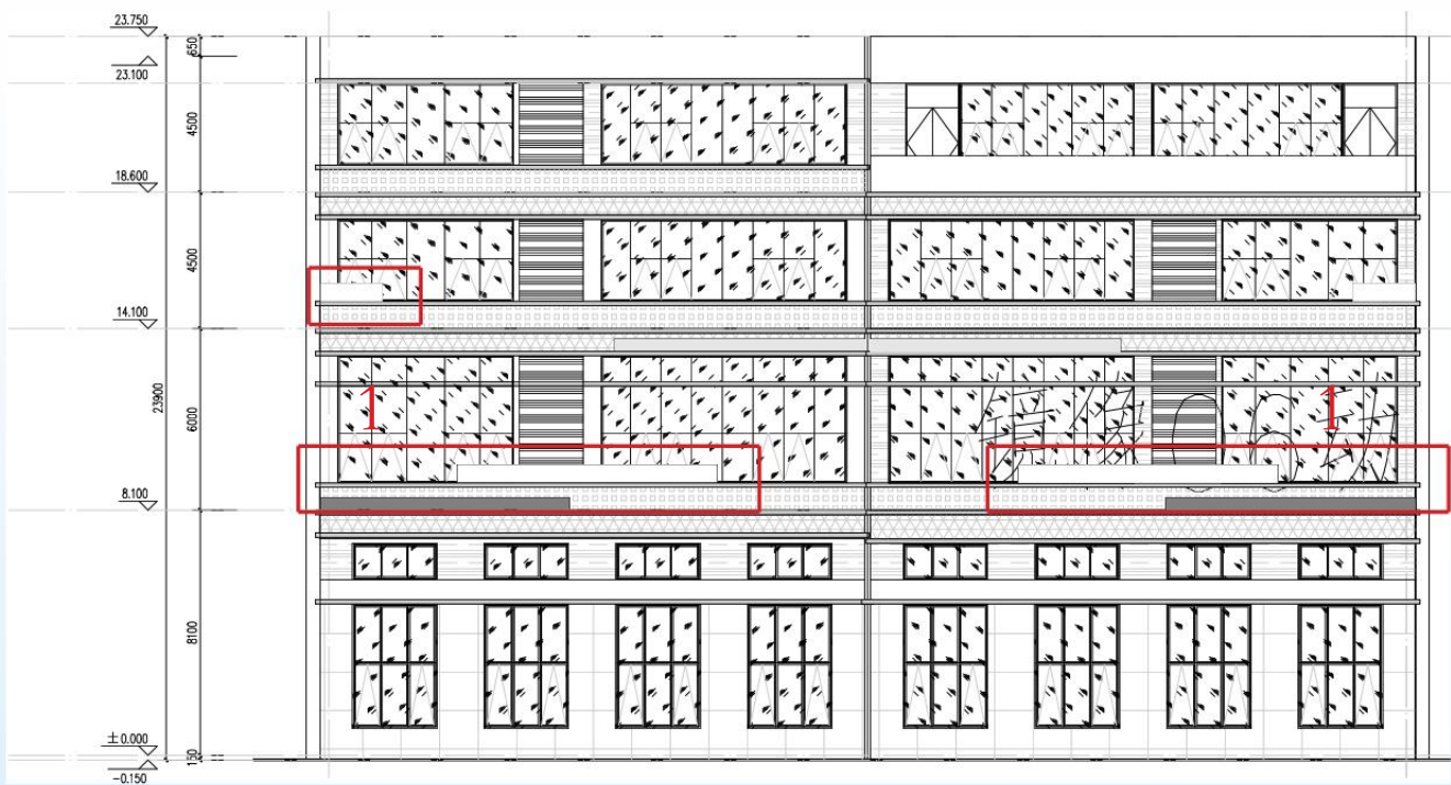
变更前 08 栋东立面图
