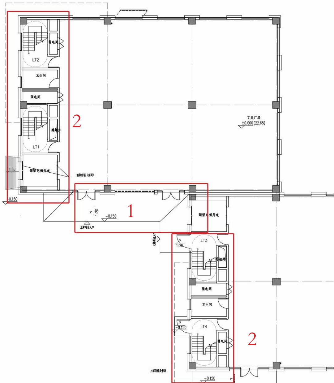
变更后 04 栋一层平面图
