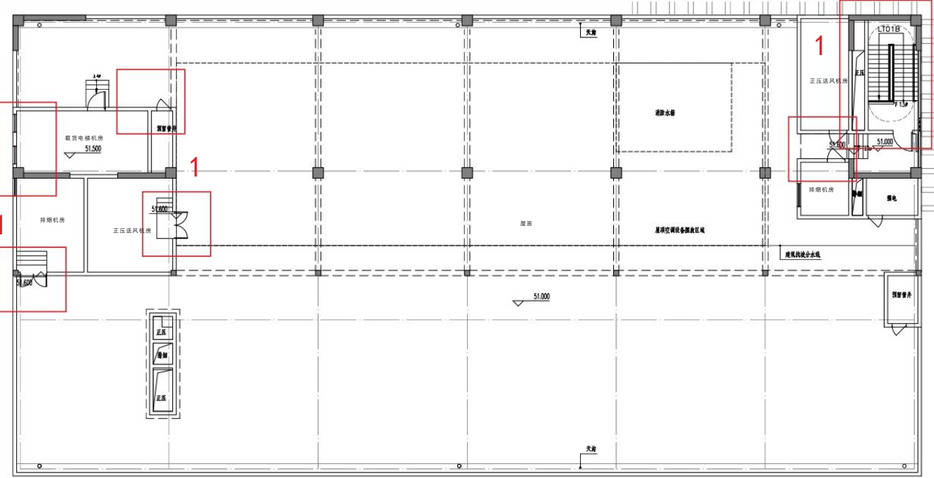
变更后 01 栋屋顶层平面图
