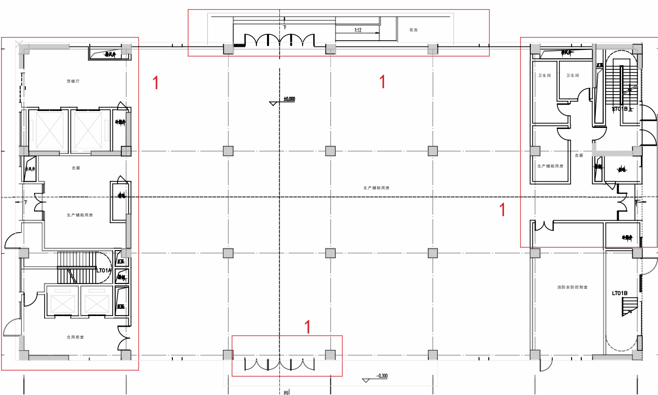
变更前 01 栋一层平面图
