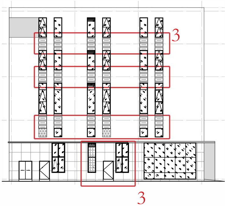
变更后 10 栋东、西立面图
