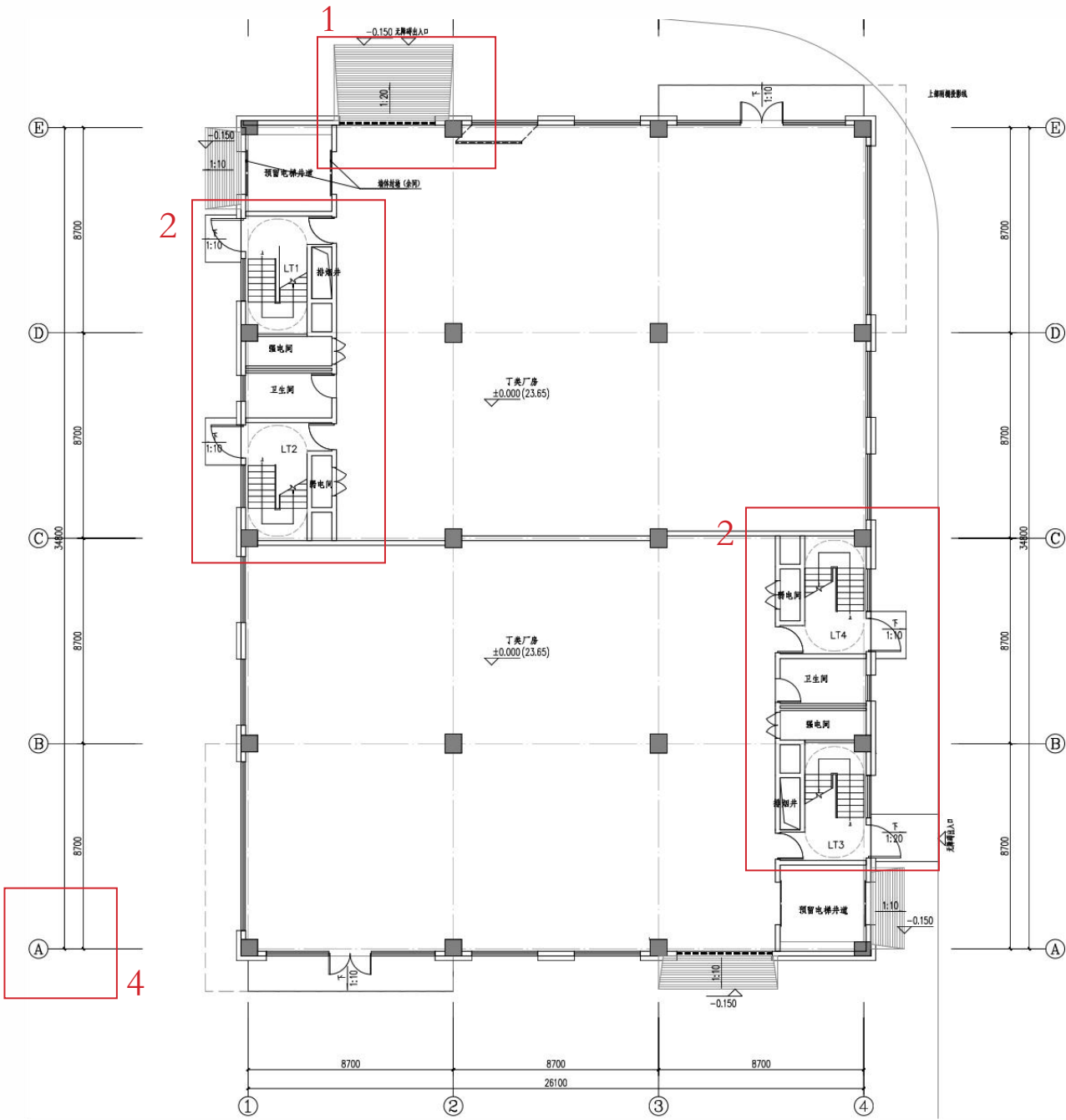
变更后 02 栋平面图（09 栋为镜像布置）
