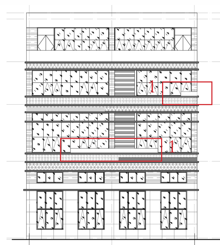
变更后 05 栋西立面图（06、07 栋为镜像布置）
