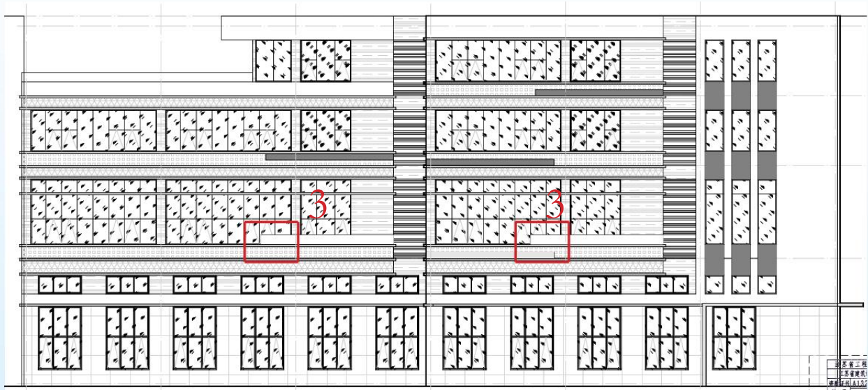
变更前 04 栋南立面图
