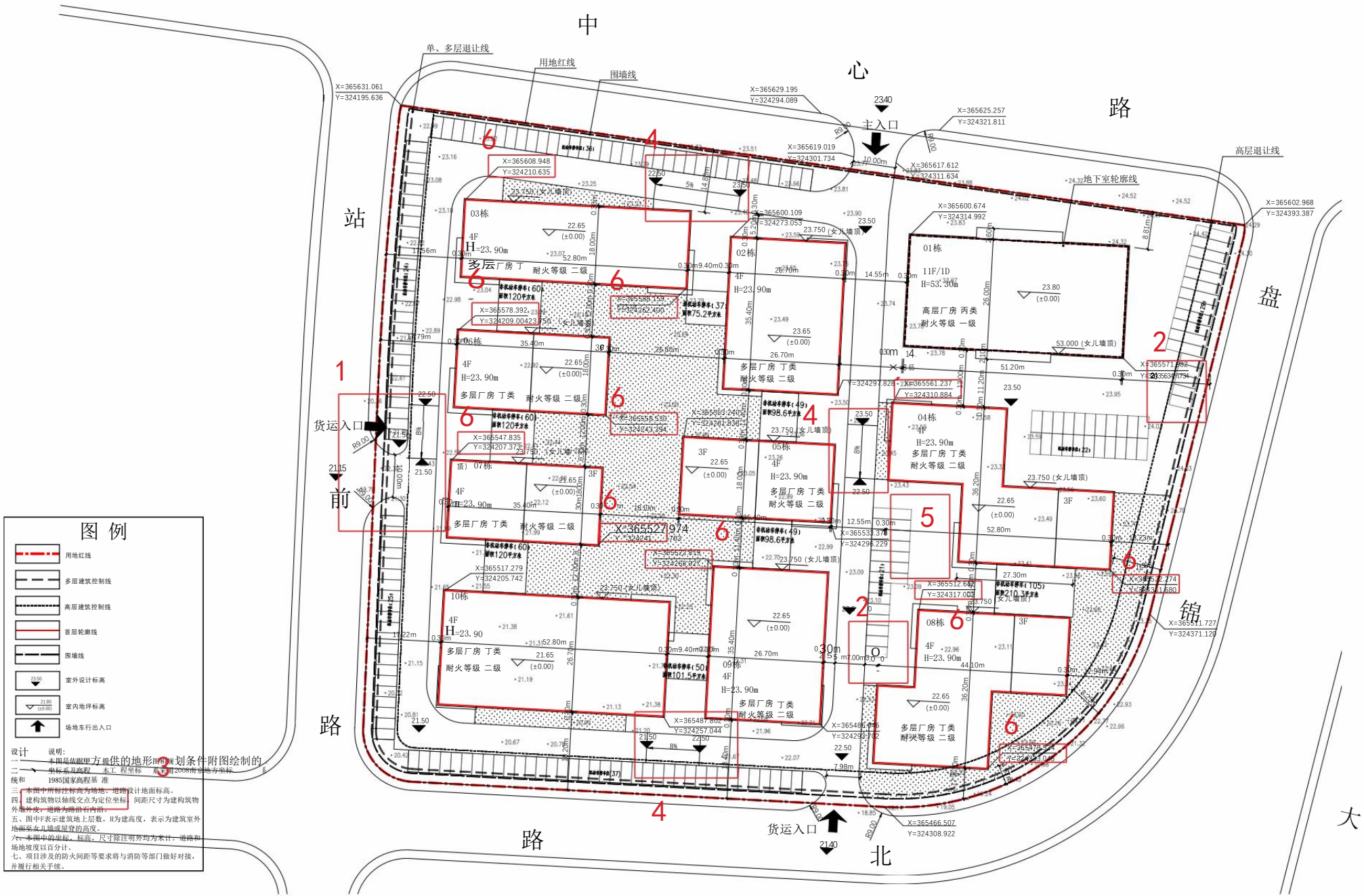
变更后 红线定位图
