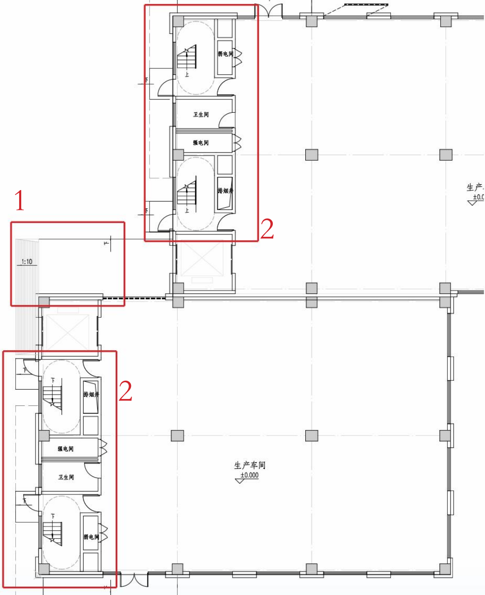
变更前 08 栋一层平面图
