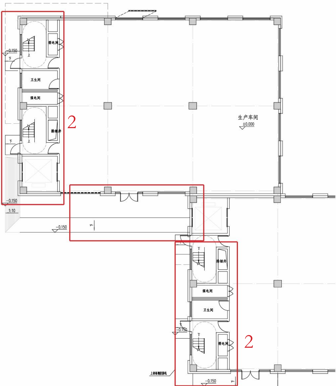
变更前 04 栋一层平面图
