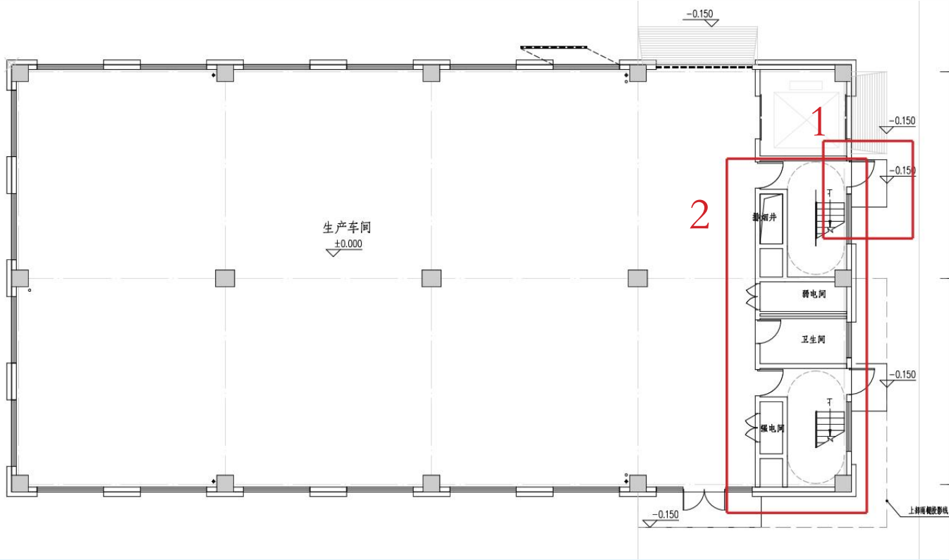
变更前 05 栋一层平面图 (06、07 栋为镜像布置)
