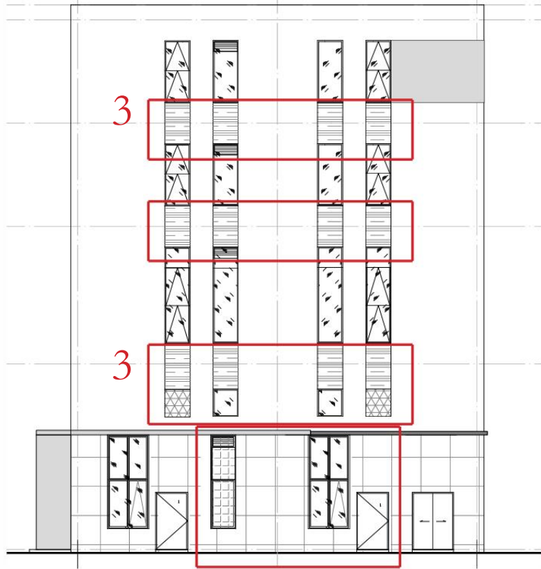
变更后 05 栋东立面图（06、07 栋为镜像布置）
