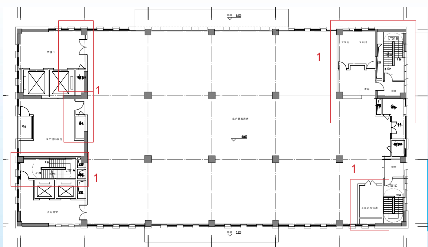
变更后 01 栋二层平面图
