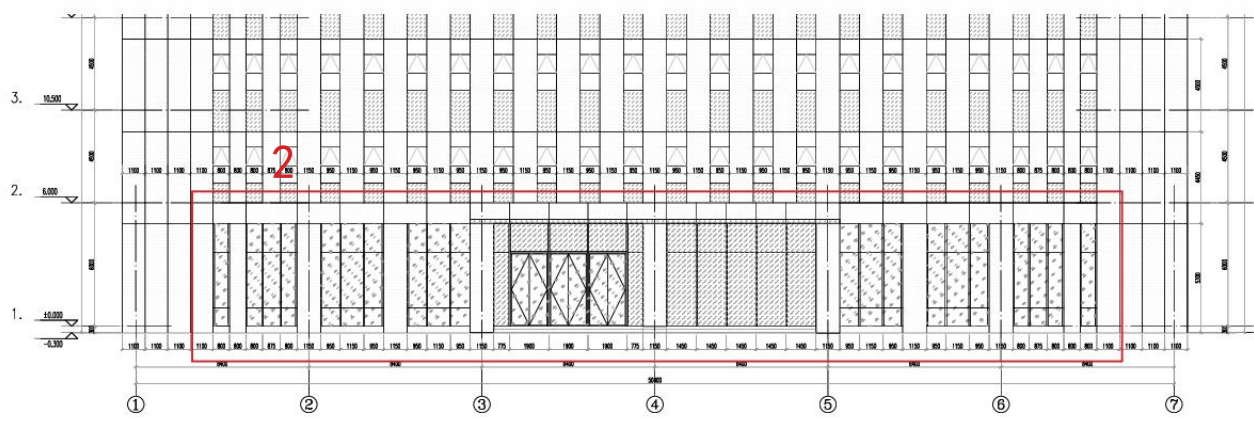
变更前 01 栋 1 轴 -7 轴立面图
