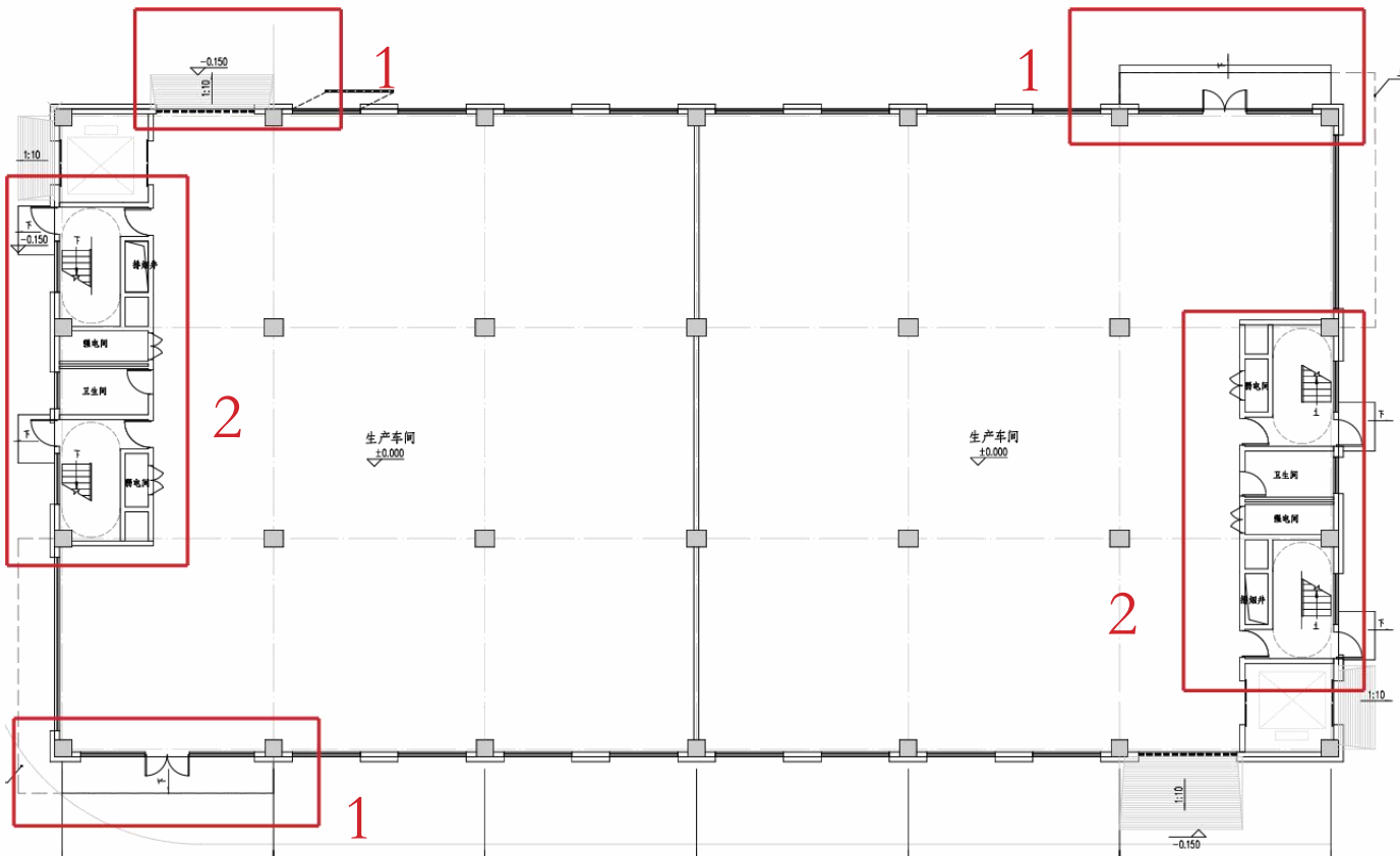
变更前 10 栋一层平面图
