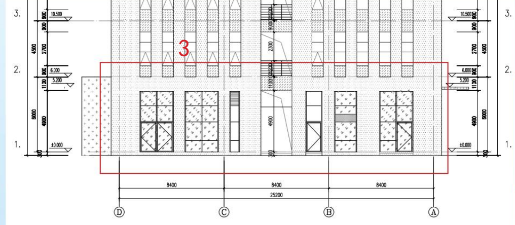
变更后 01 栋 1 轴 -7 轴立面图
