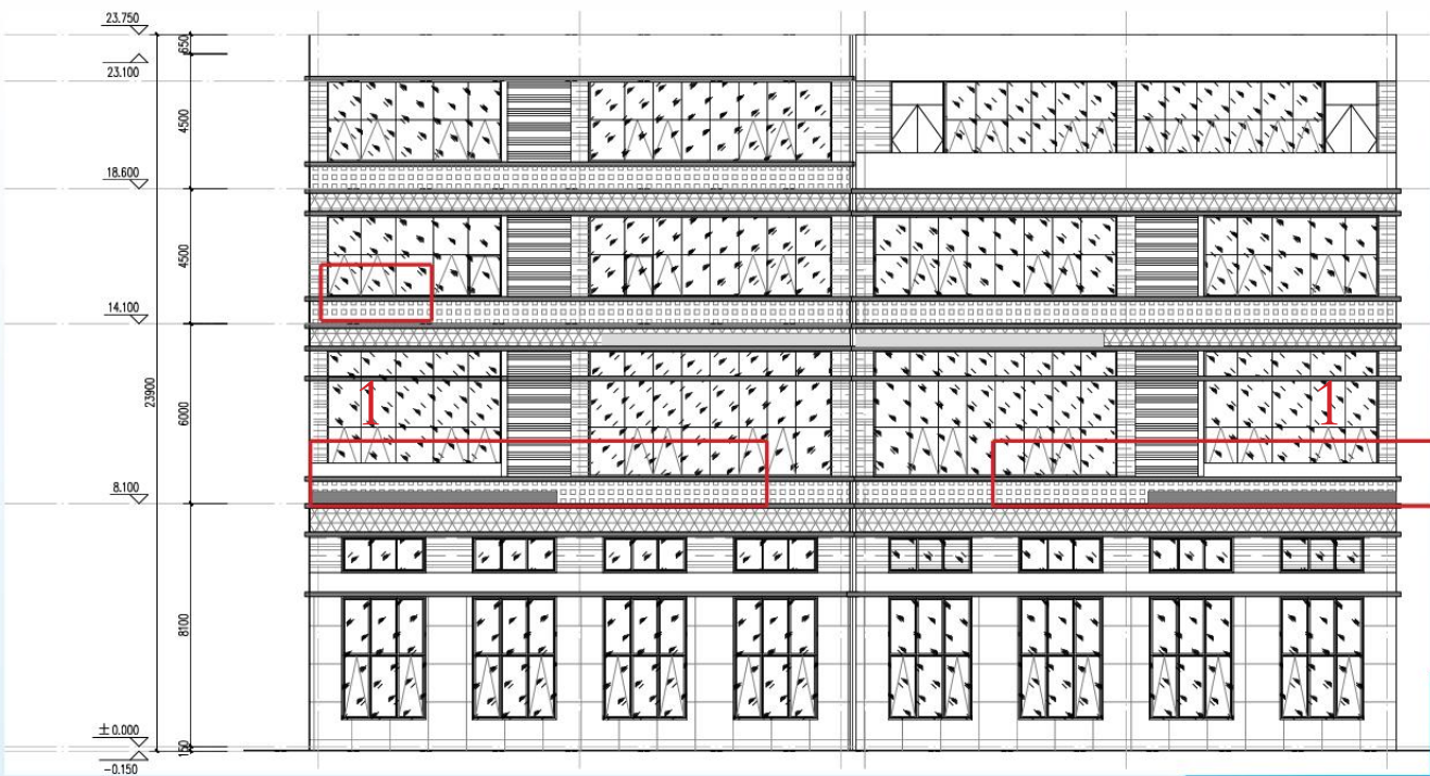
变更后 08 栋东立面图
