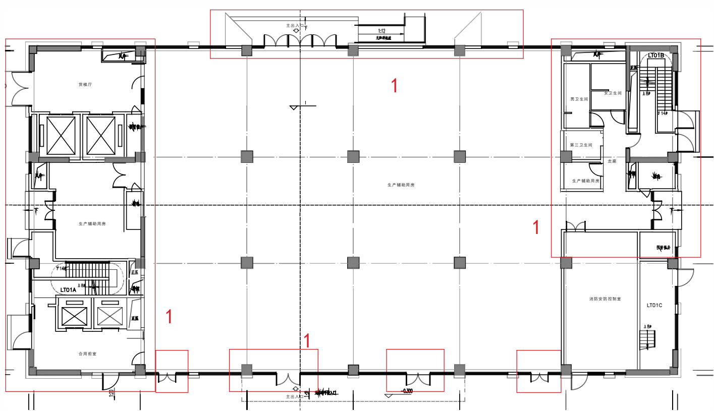
变更后 01 栋一层平面图
