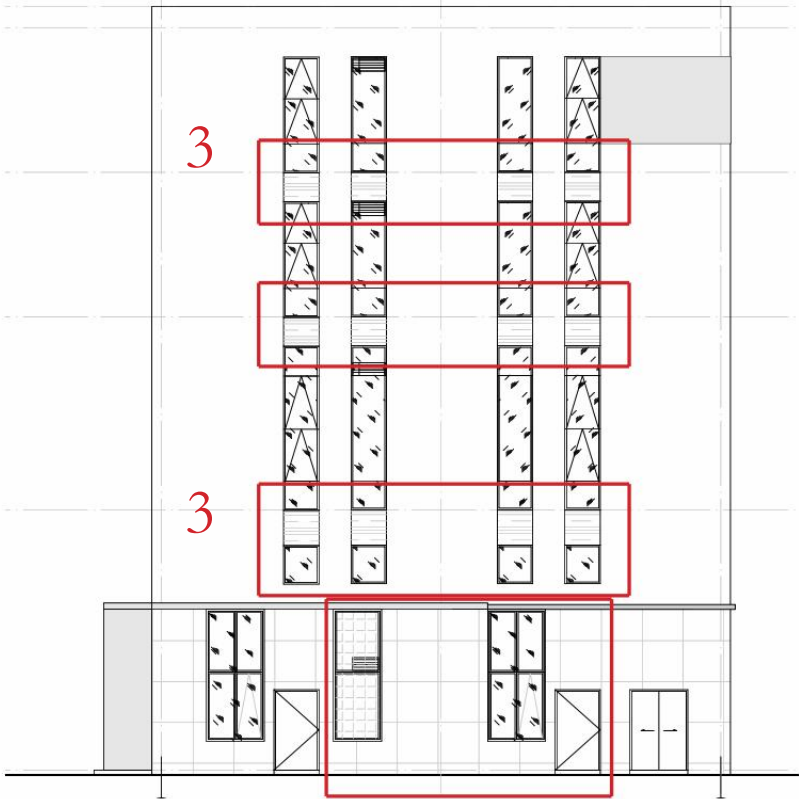
变更前 05 栋东立面图（06、07 栋为镜像布置）
