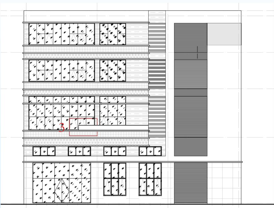
变更后 02 栋南、北立面图（09 栋为镜像布置）
