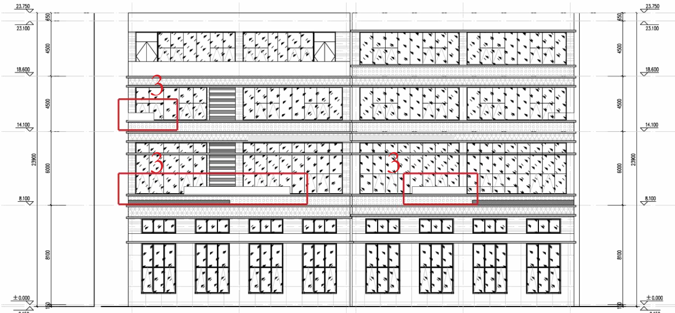
变更前 04 栋东立面图
