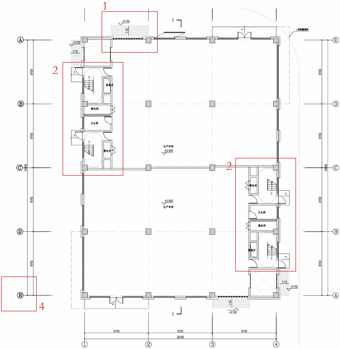
变更前 02 栋平面图（09 栋为镜像布置）
