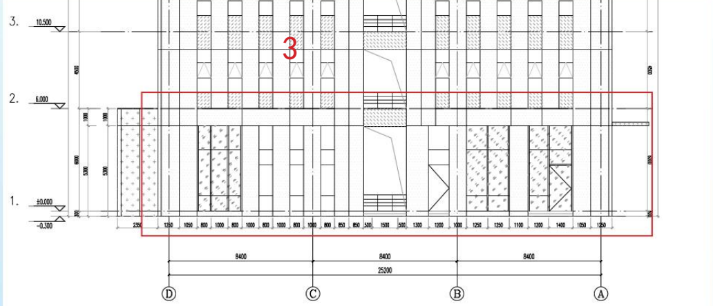
变更前 01 栋 1 轴 -7 轴立面图
