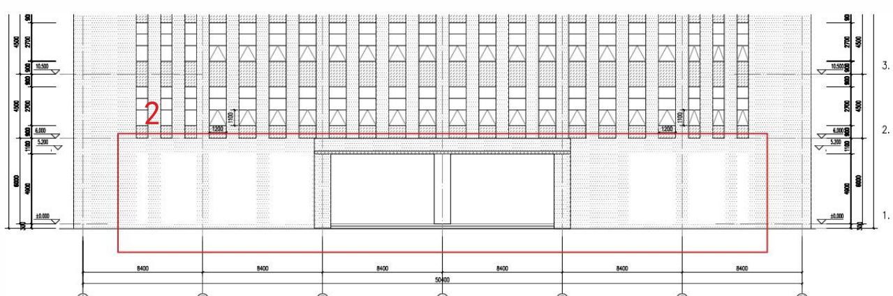
变更后 01 栋 1 轴 -7 轴立面图
