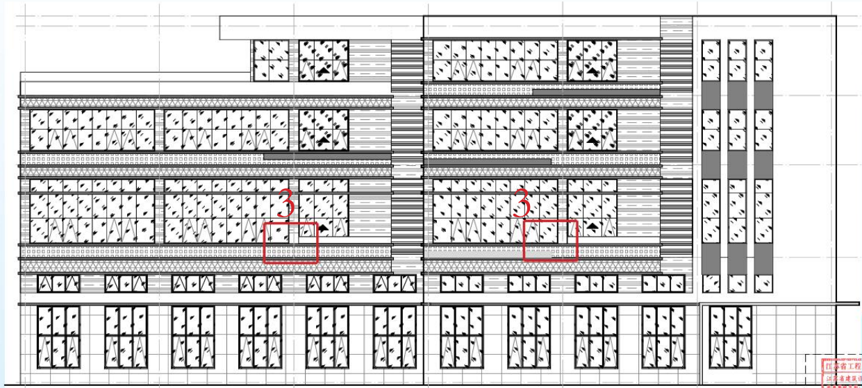
变更后 04 栋南立面图
