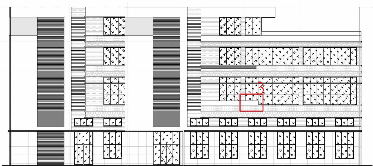
变更前 04 栋北立面图
