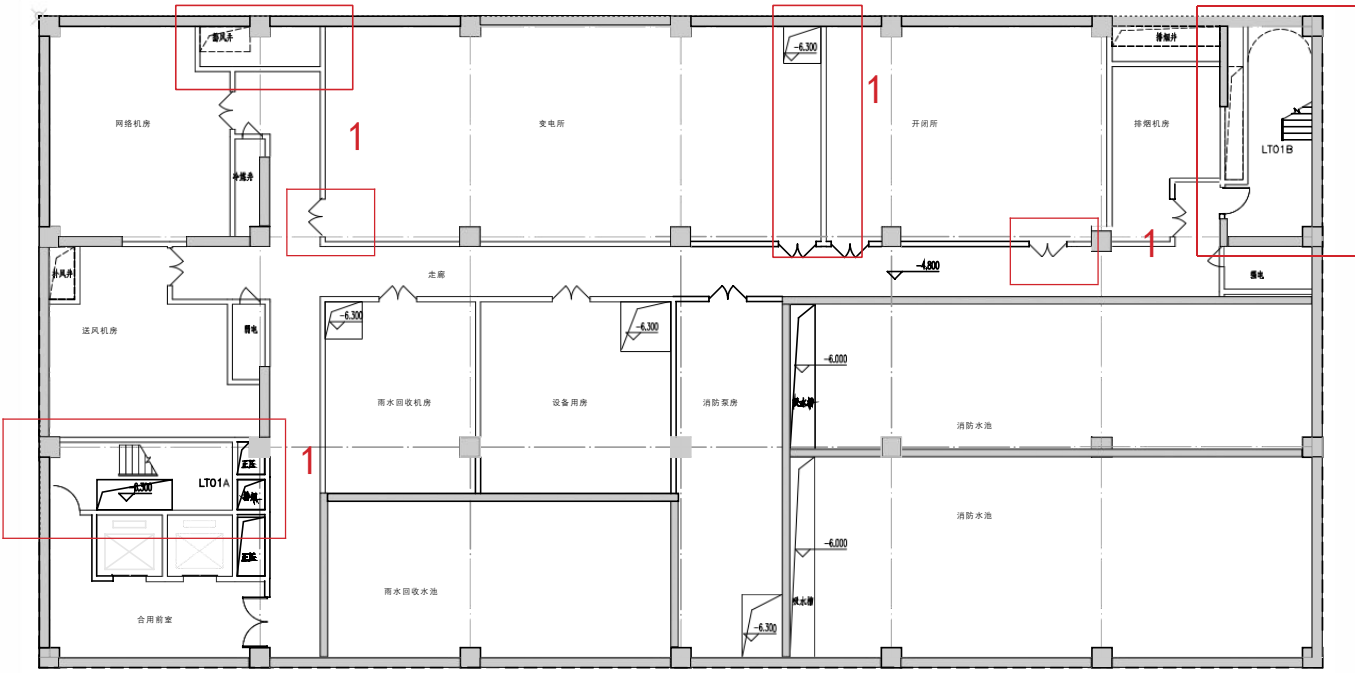
变更前 01 栋地下一层平面图
