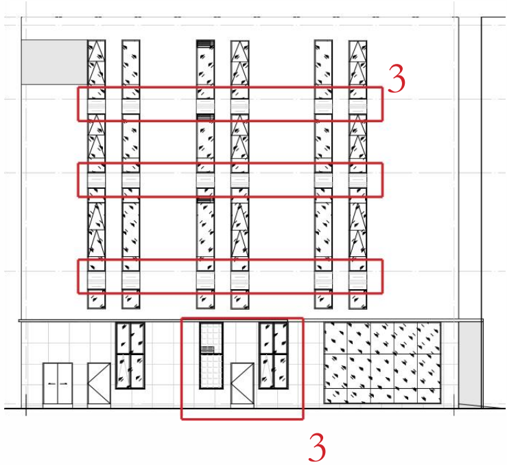
变更前 10 栋东、西立面图
