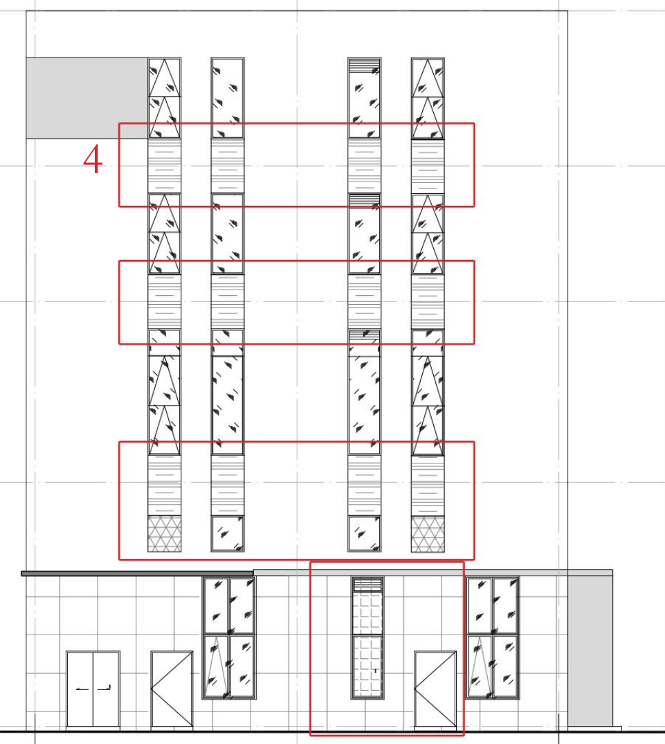
变更后 03 栋西立面图、东立面图
