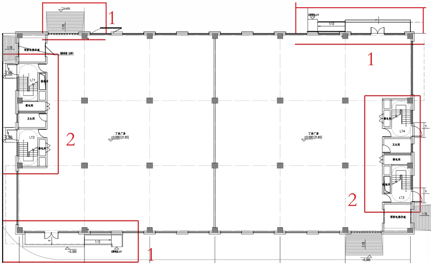
变更后 10 栋一层平面图
