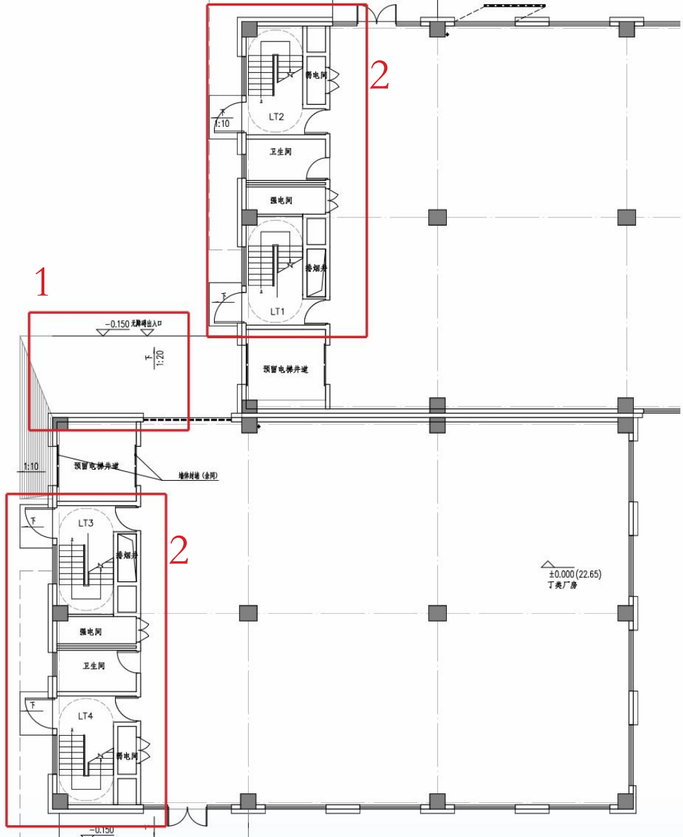
变更后 08 栋一层平面图
