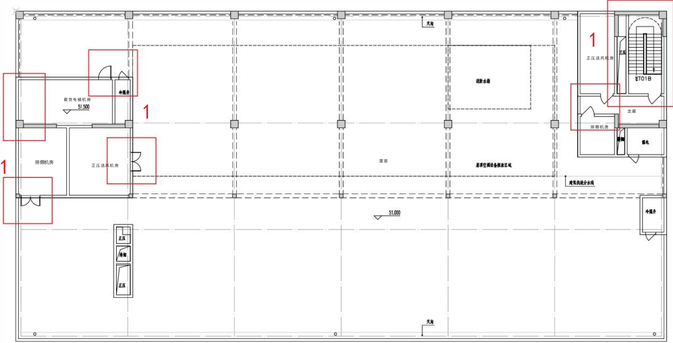
变更前 01 栋屋顶层平面图
