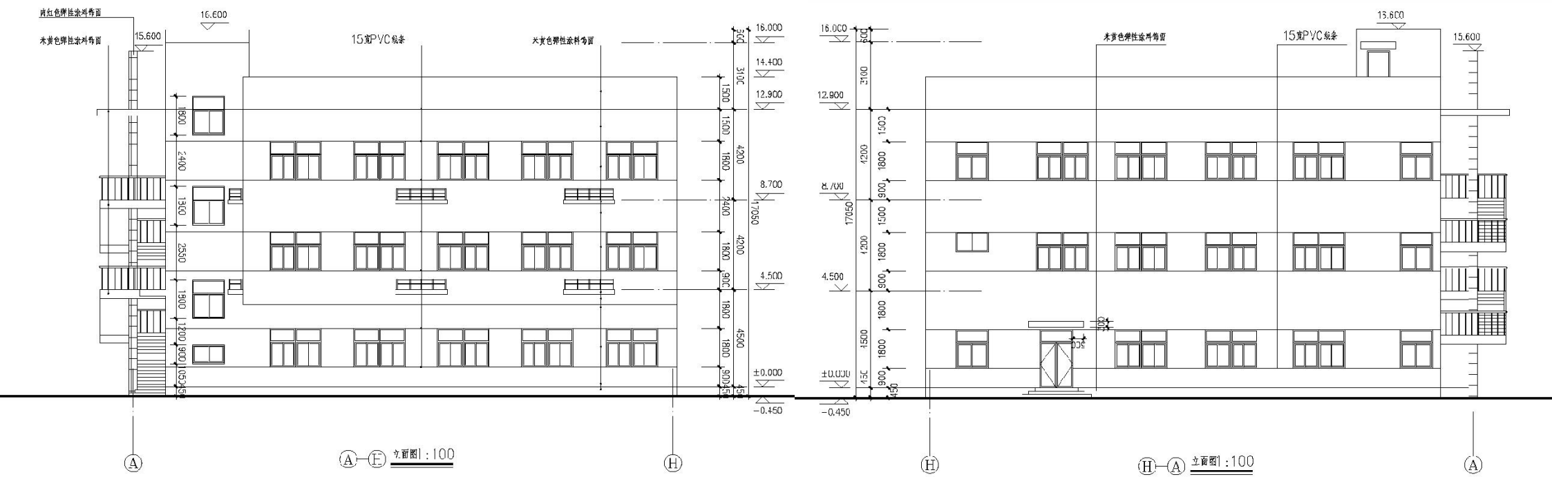
变更后服务楼 A-H、H-A 立面图：
