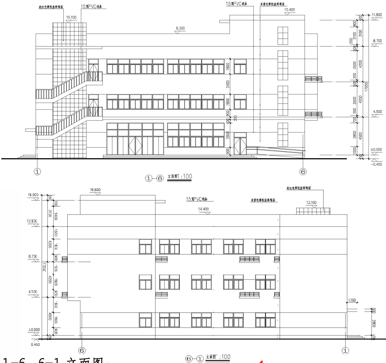
变更前服务楼 1-6、6-1 立面图：
