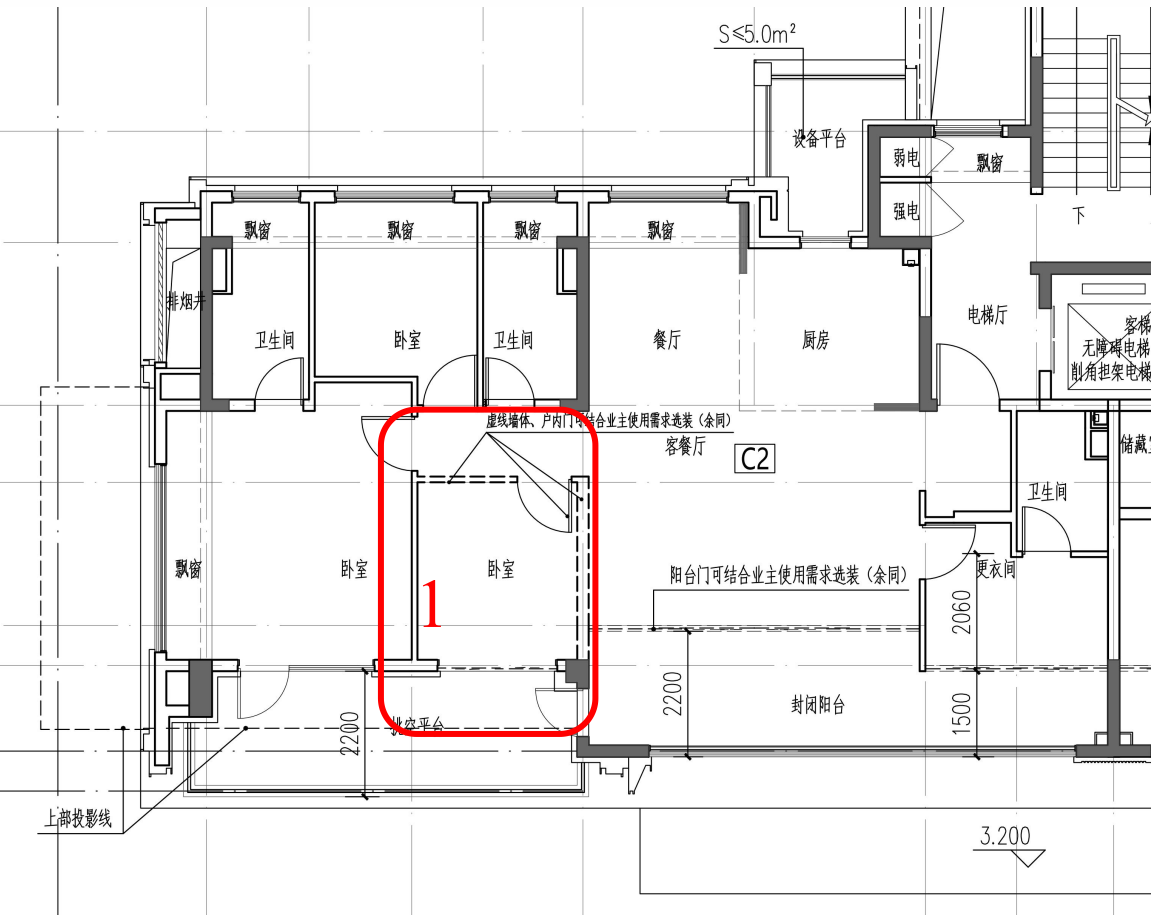
C2 户型平面图
