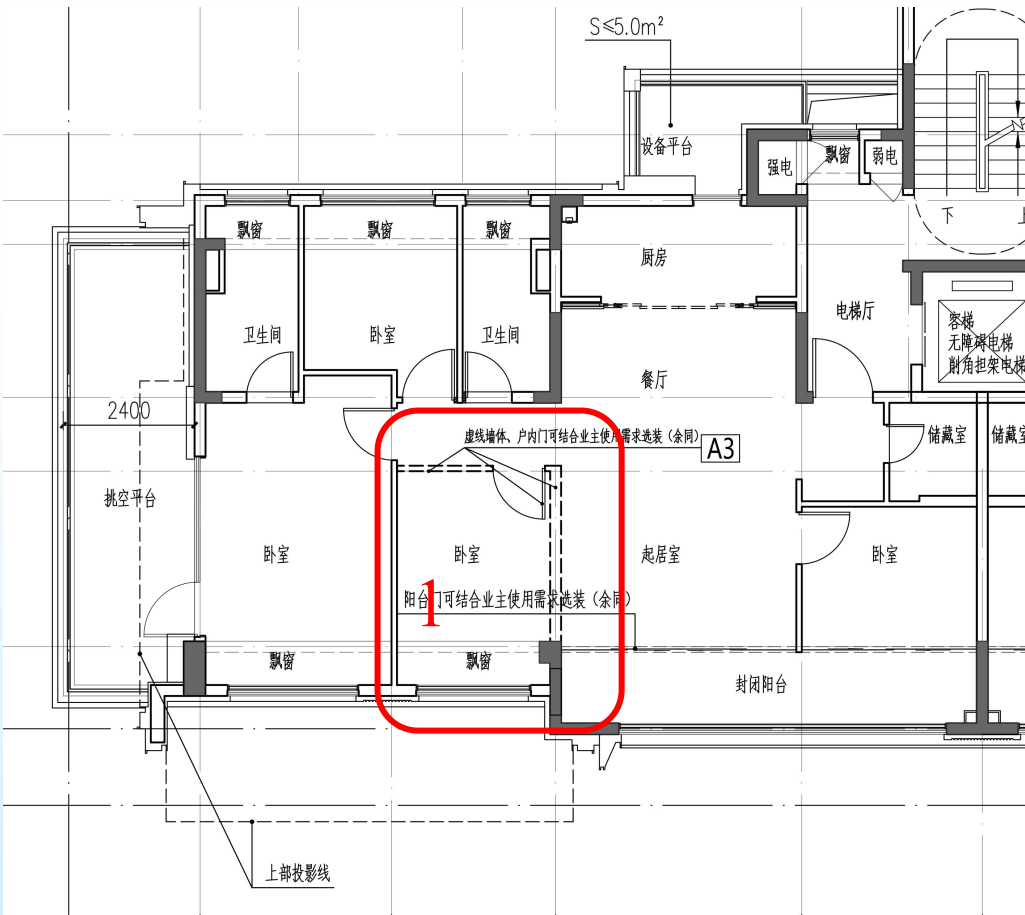
A3 户型平面图
