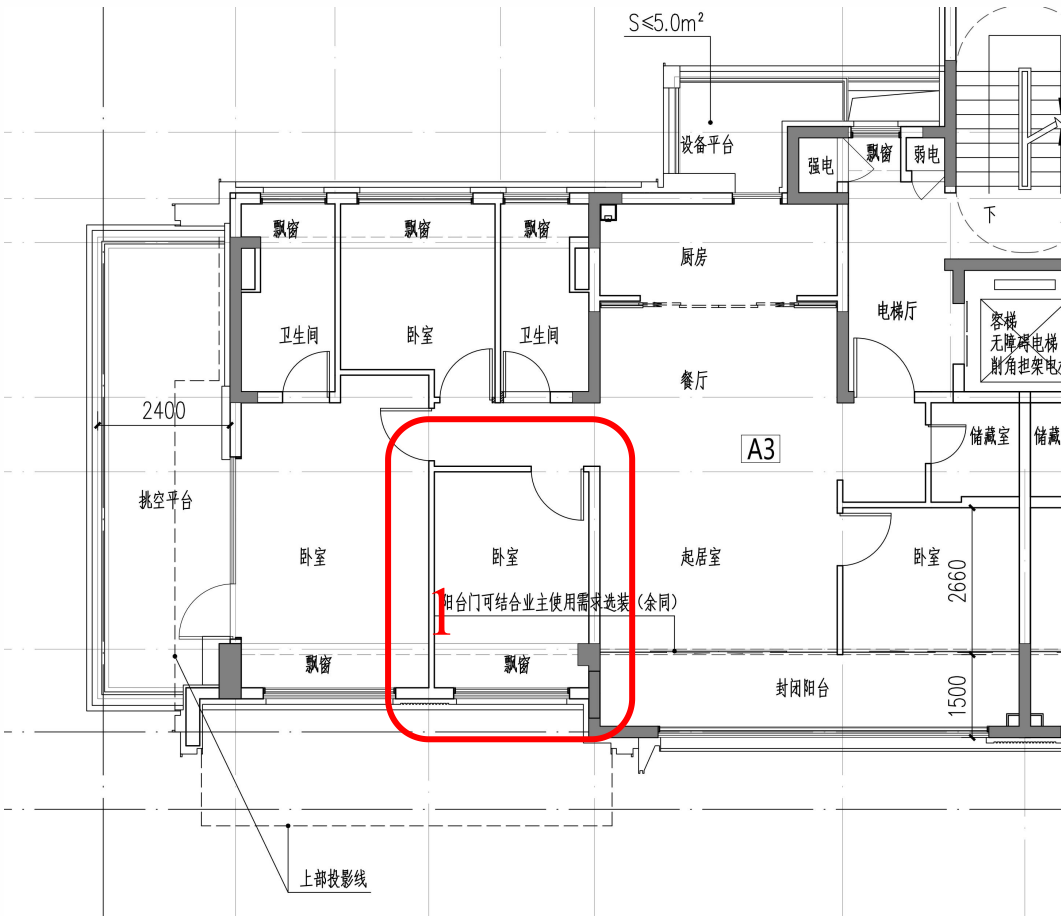
A3 户型平面图
