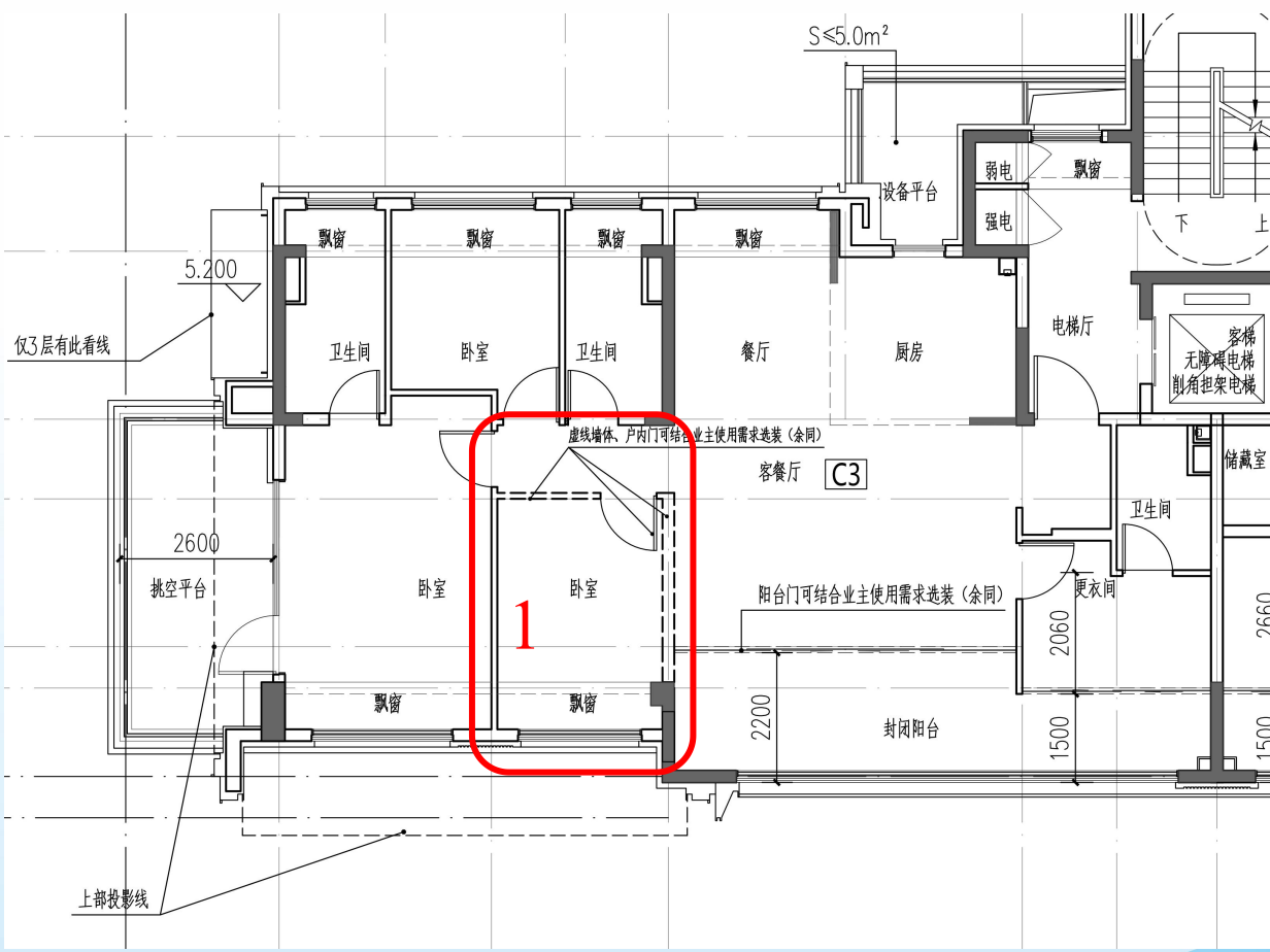
C3 户型平面图
