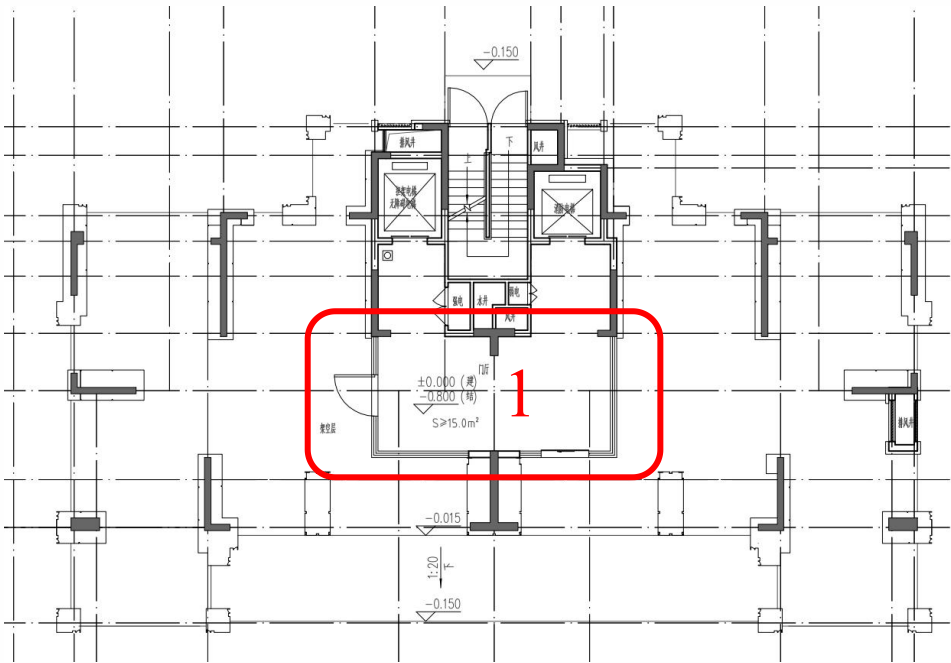
10# 一层平面图
