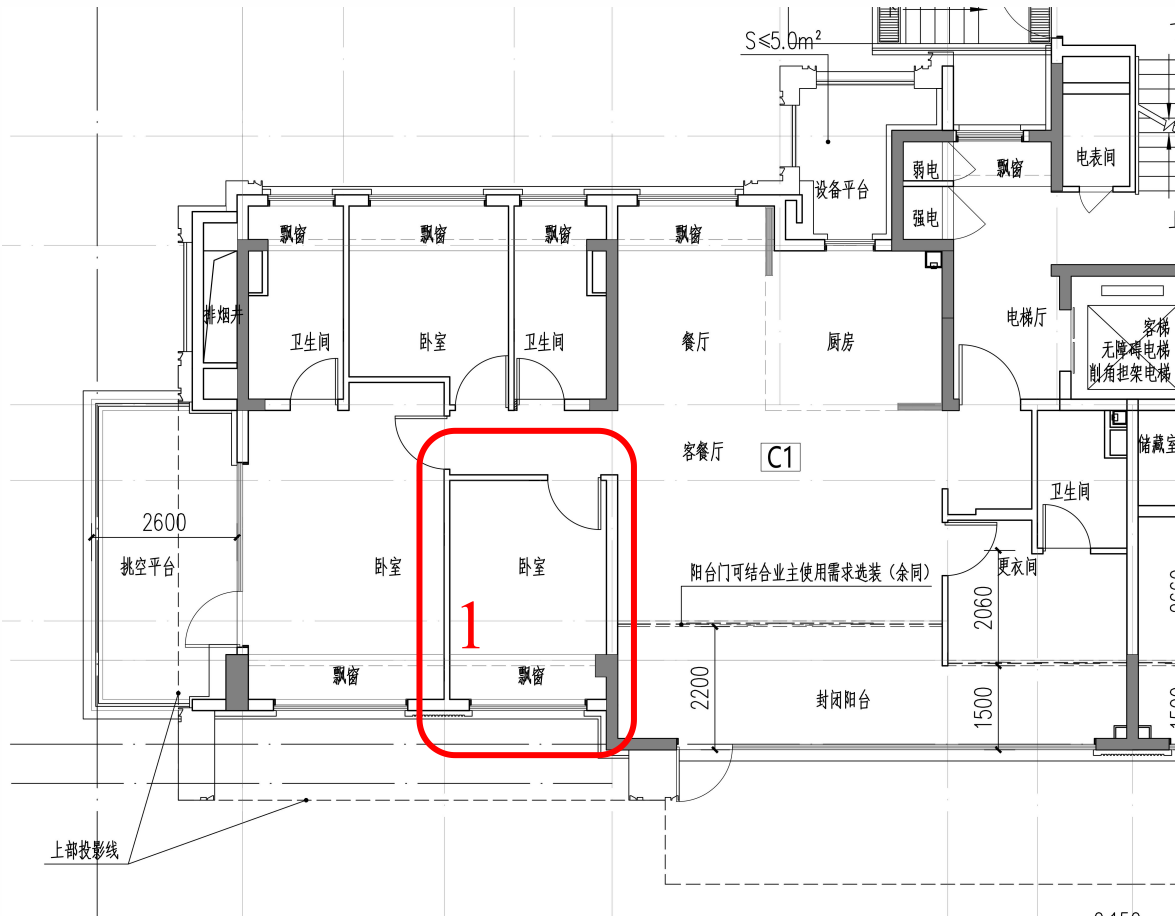
C1 户型平面图
