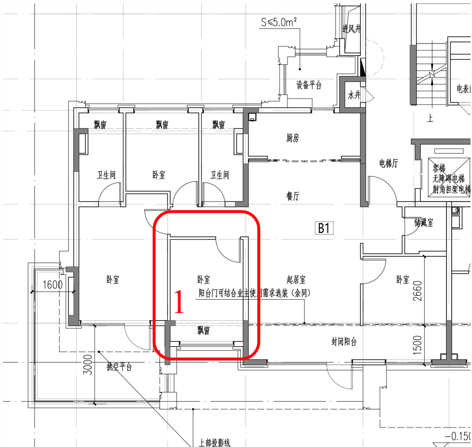
B1 户型平面图
