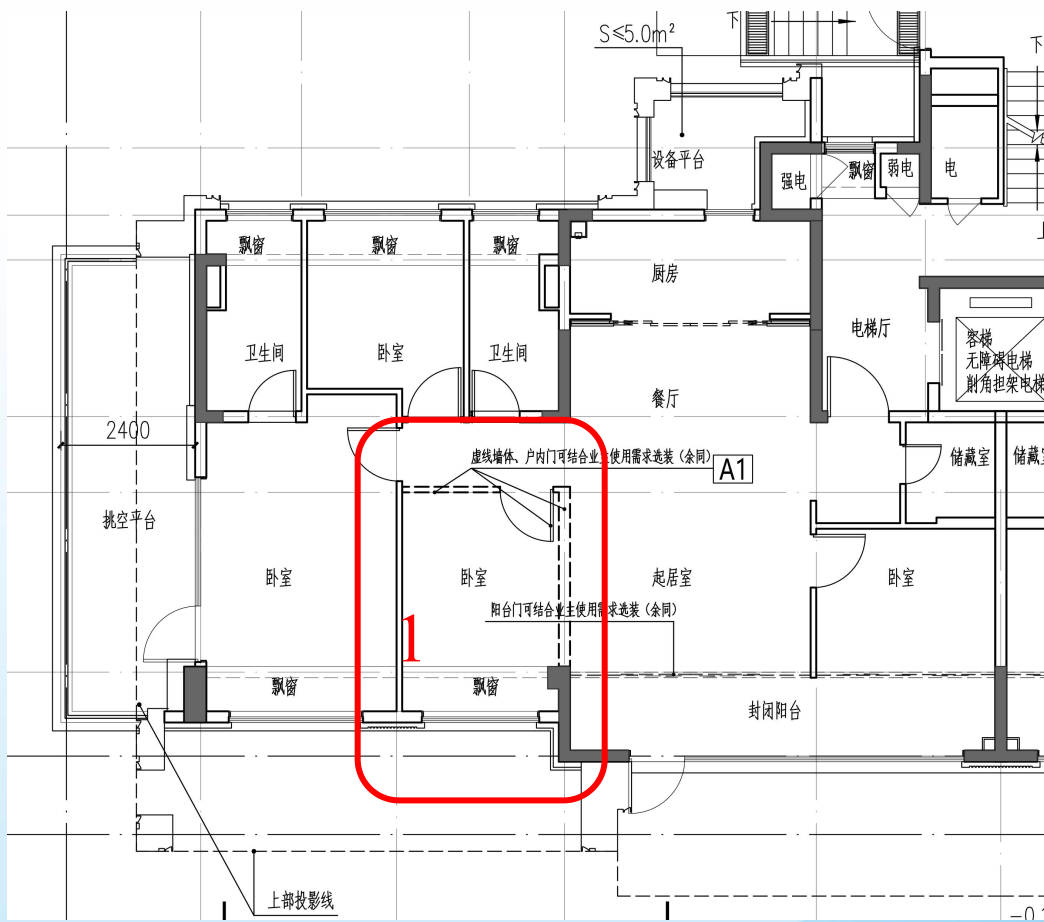
A1 户型平面图
