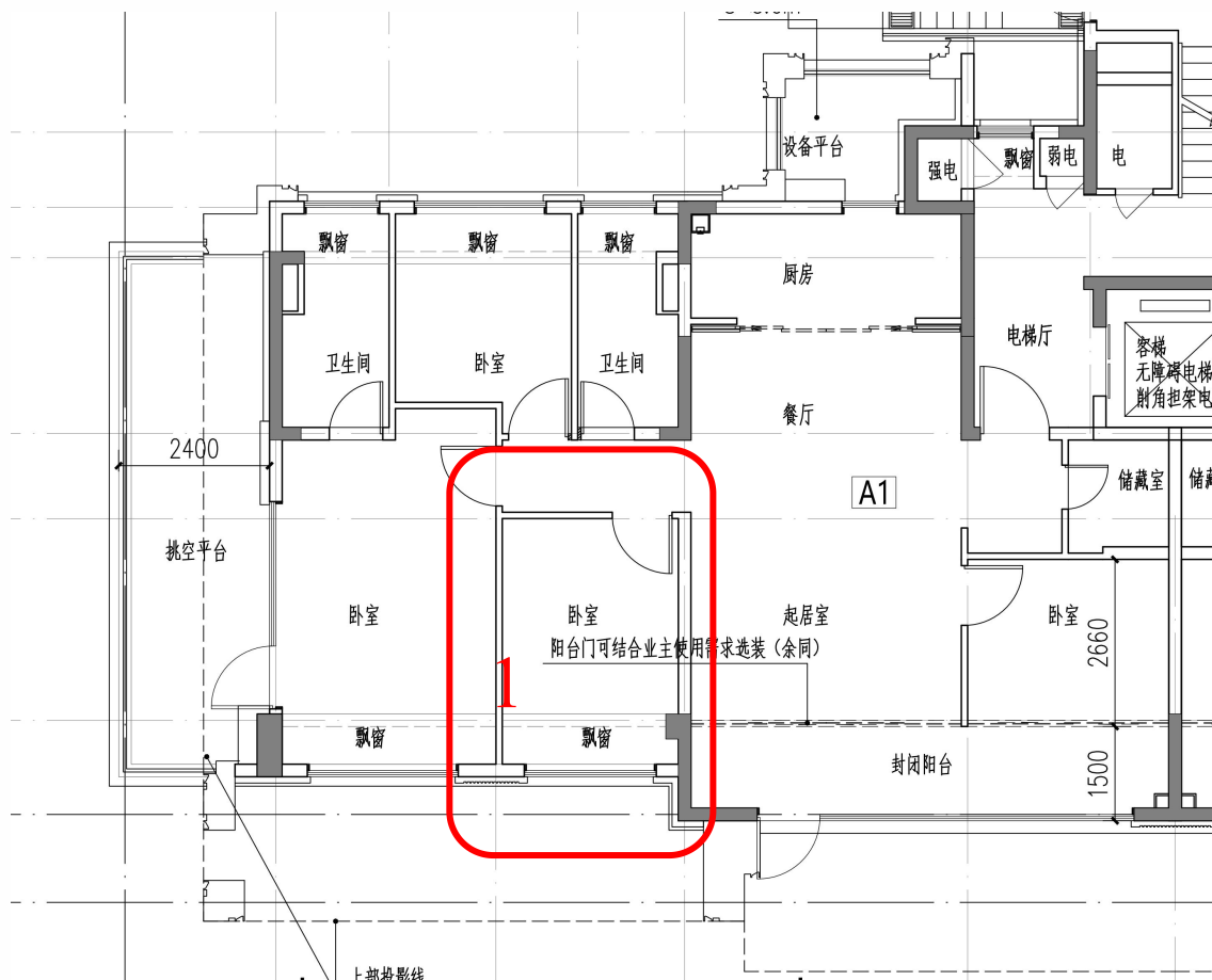
A1 户型平面图
