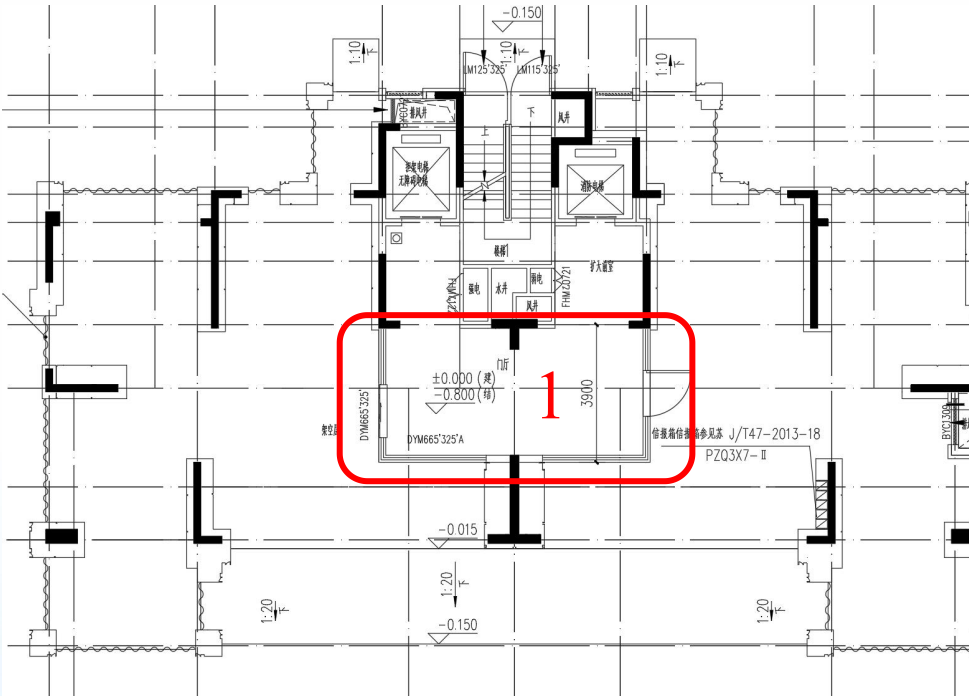
10# 一层平面图
