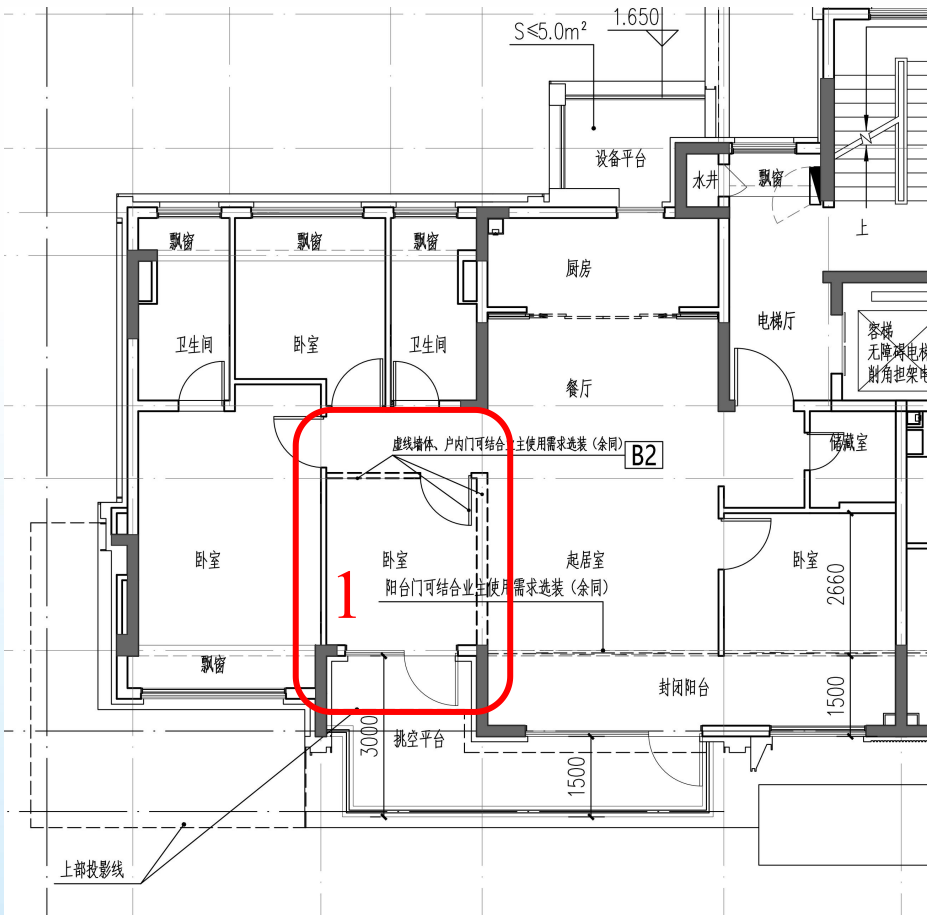
B2 户型平面图
