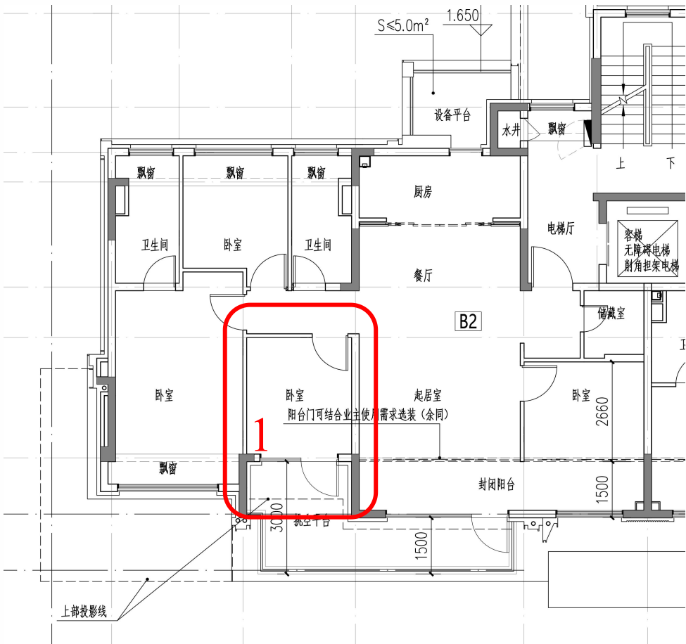
B2 户型平面图
