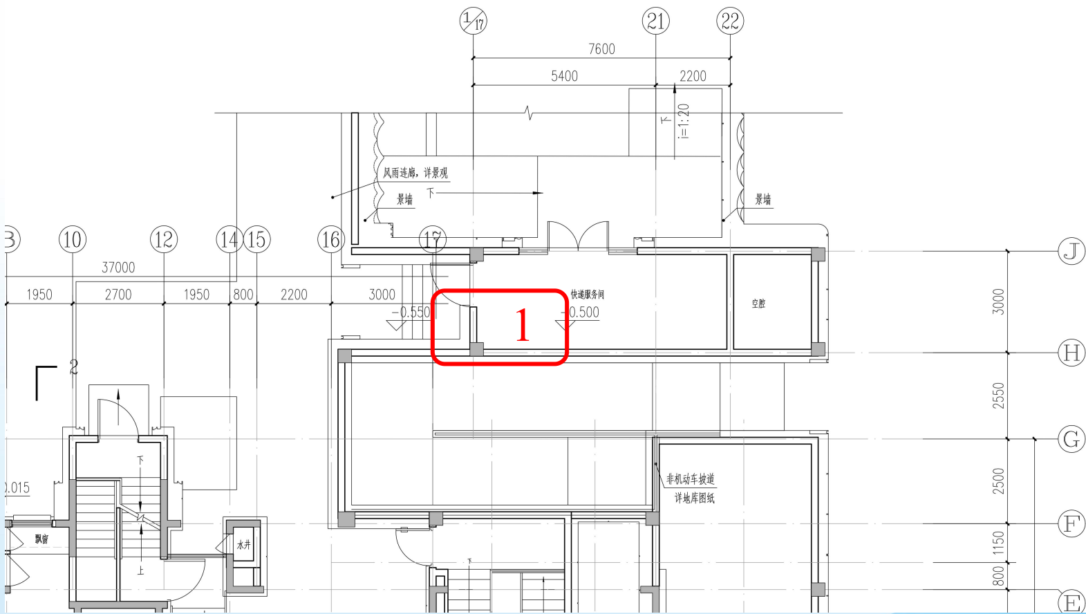
5# 一层平面图
