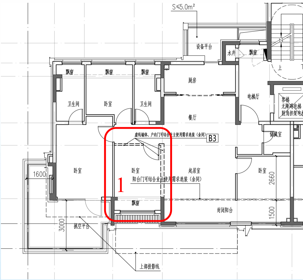
B3 户型平面图
