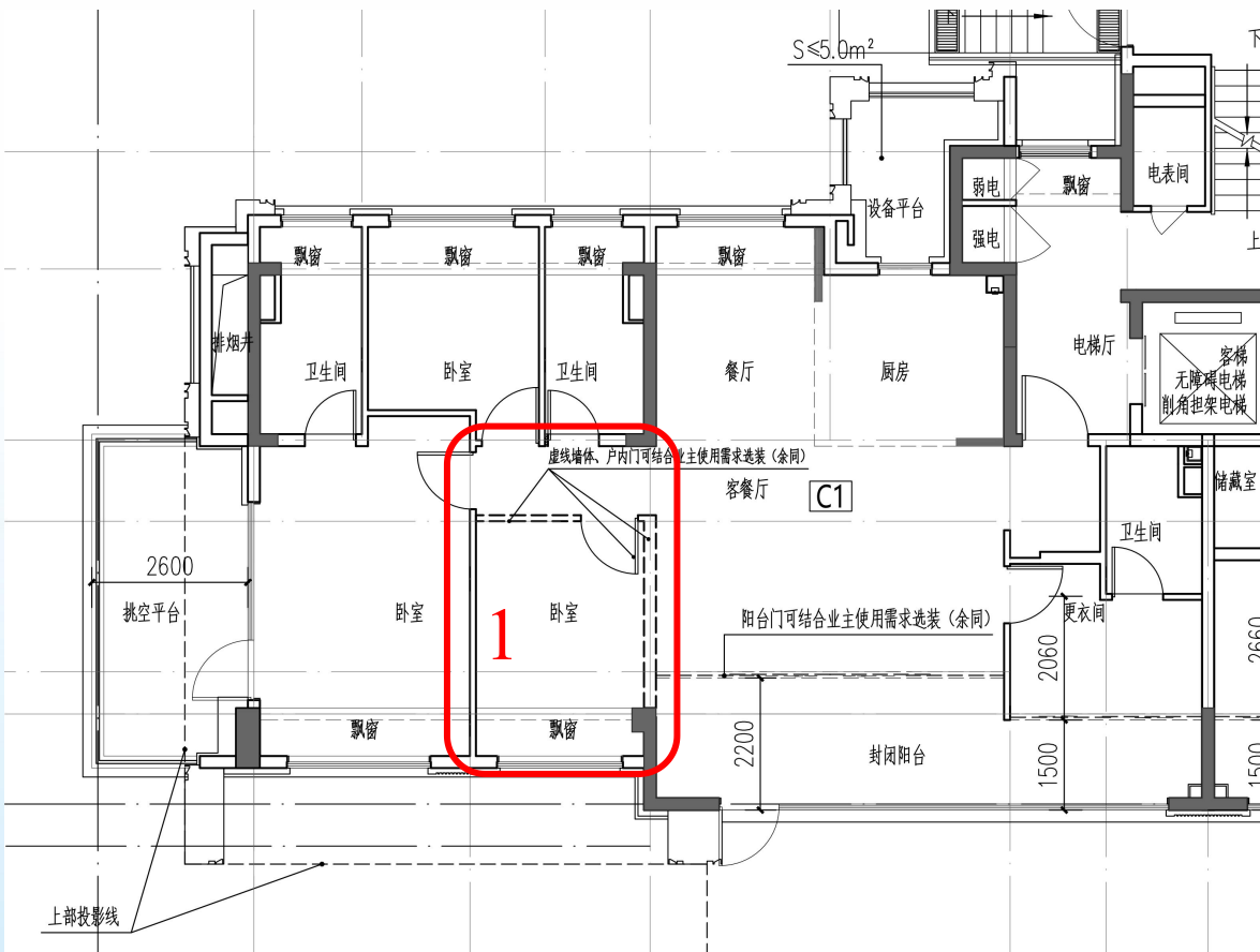
C1 户型平面图
