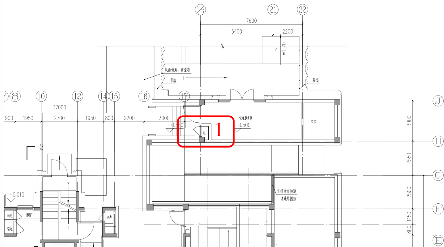
5# 一层平面图
