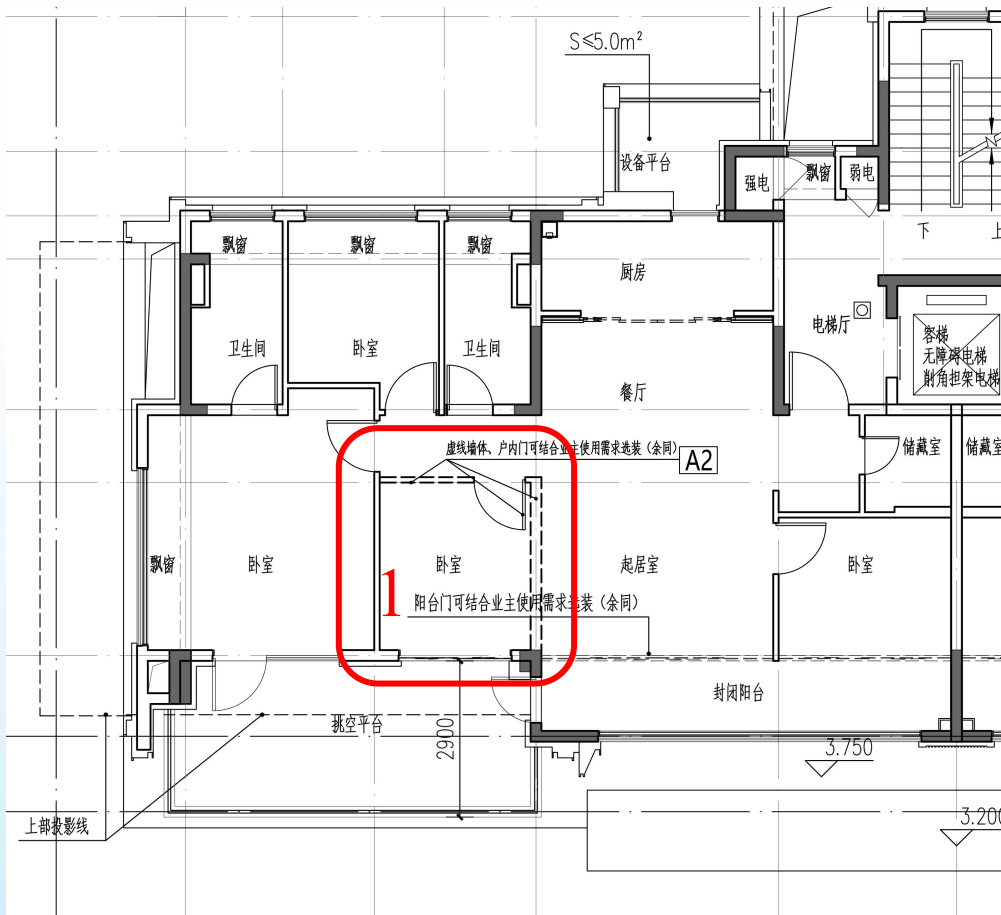
A2 户型平面图
