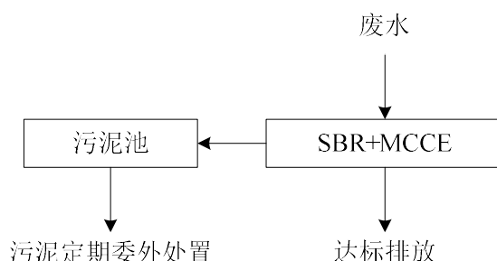
图 4-2 化学之光污水处理站废水处理工艺流程图
