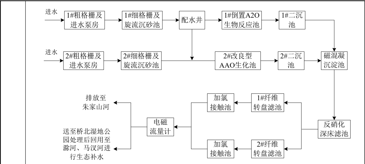
图 4-3 盘城污水处理厂工艺流程图
