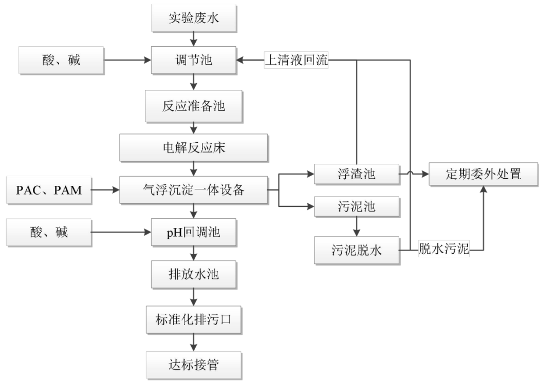
图 4-1 鼎业百泰生物大楼污水处理站废水处理工艺流程图
