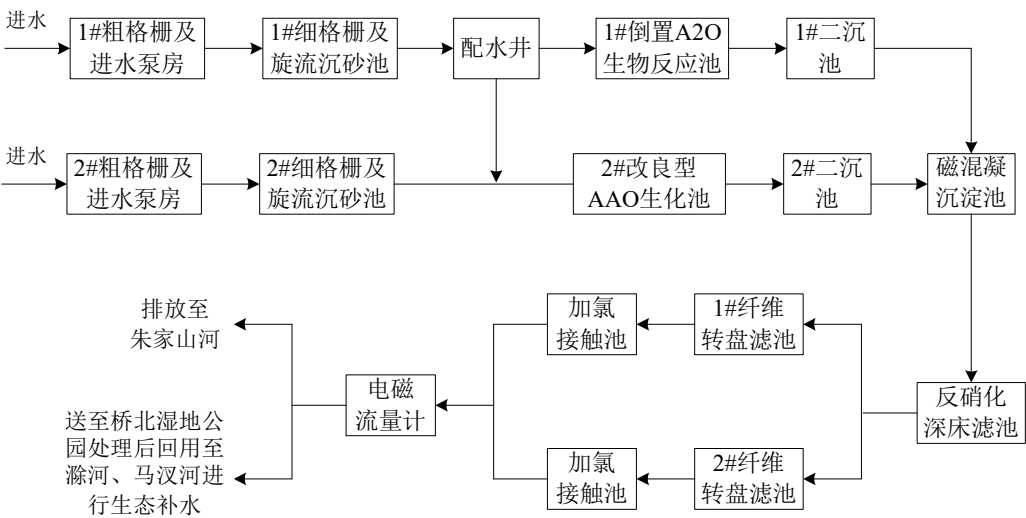
图 4-2 盘城污水处理厂工艺流程图
