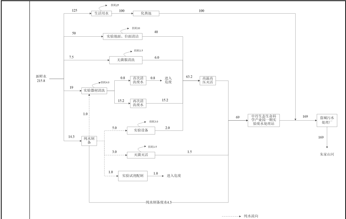
图 2-1 本项目水平衡图（单位：m³/a）
