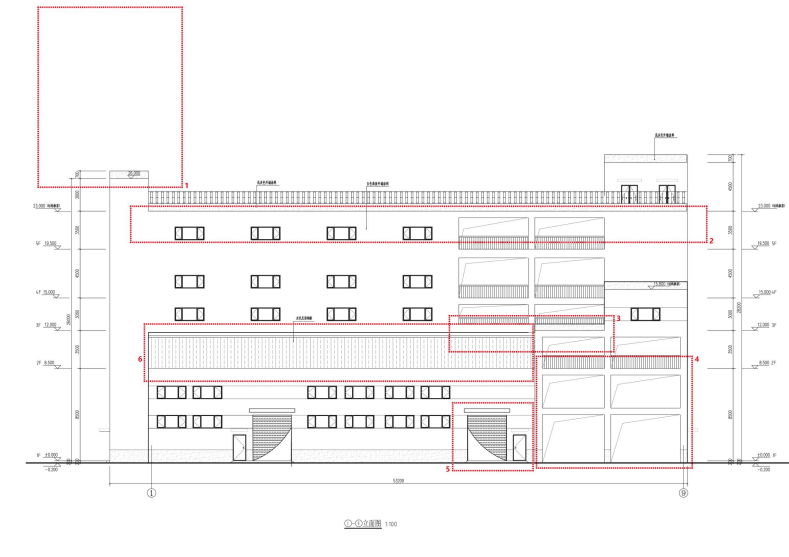
1-9 轴立面图变更后
