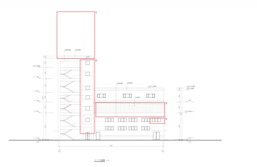
G-A 轴立面图变更后
