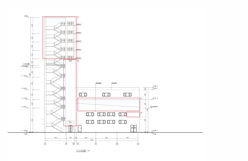
G-A 轴立面图变更前
