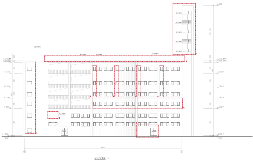
9-1 轴立面图变更前
