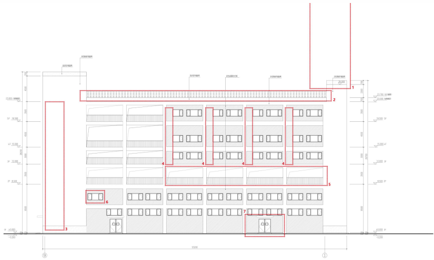
9-1 轴立面图变更后
