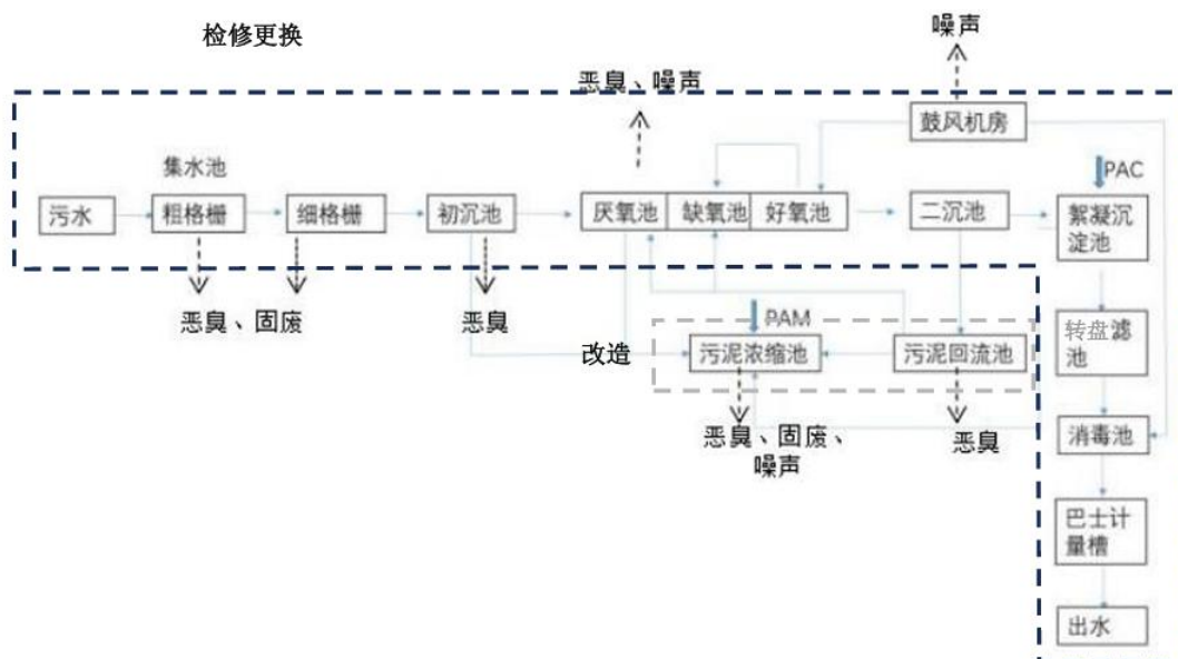
图 4-2 浦口区永宁污水处理厂处理工艺流程图
