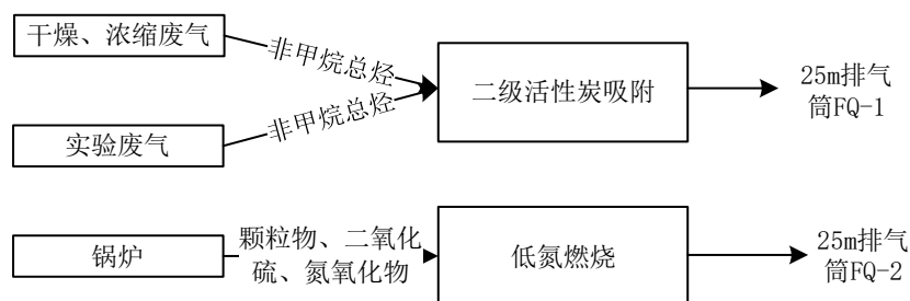
图 4-1 全厂废气处理工艺图
