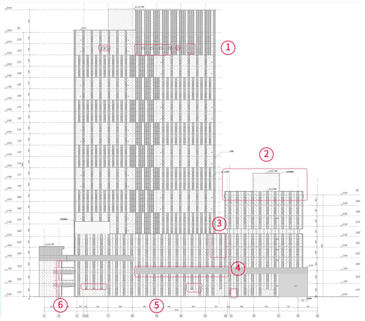
南立面图变更后
