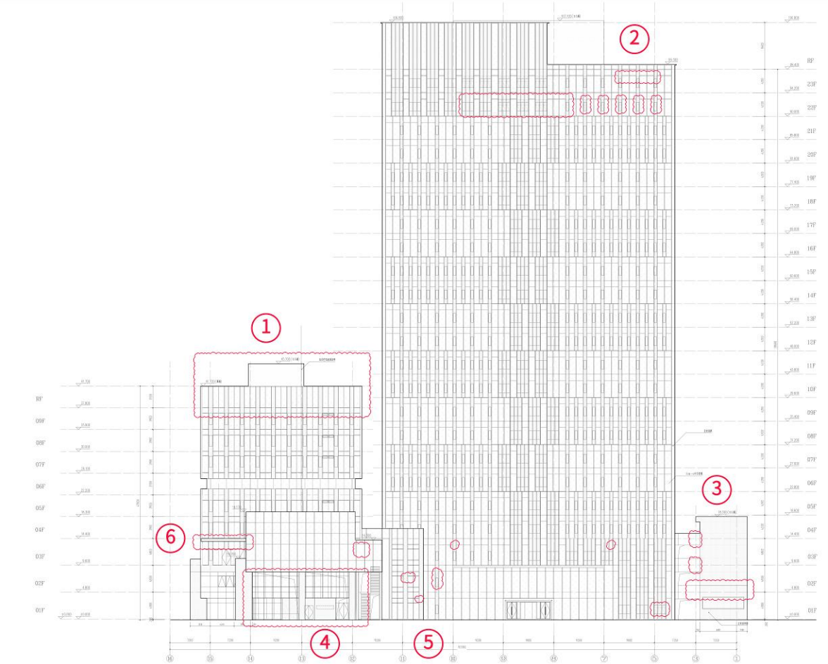
北立面图变更后
