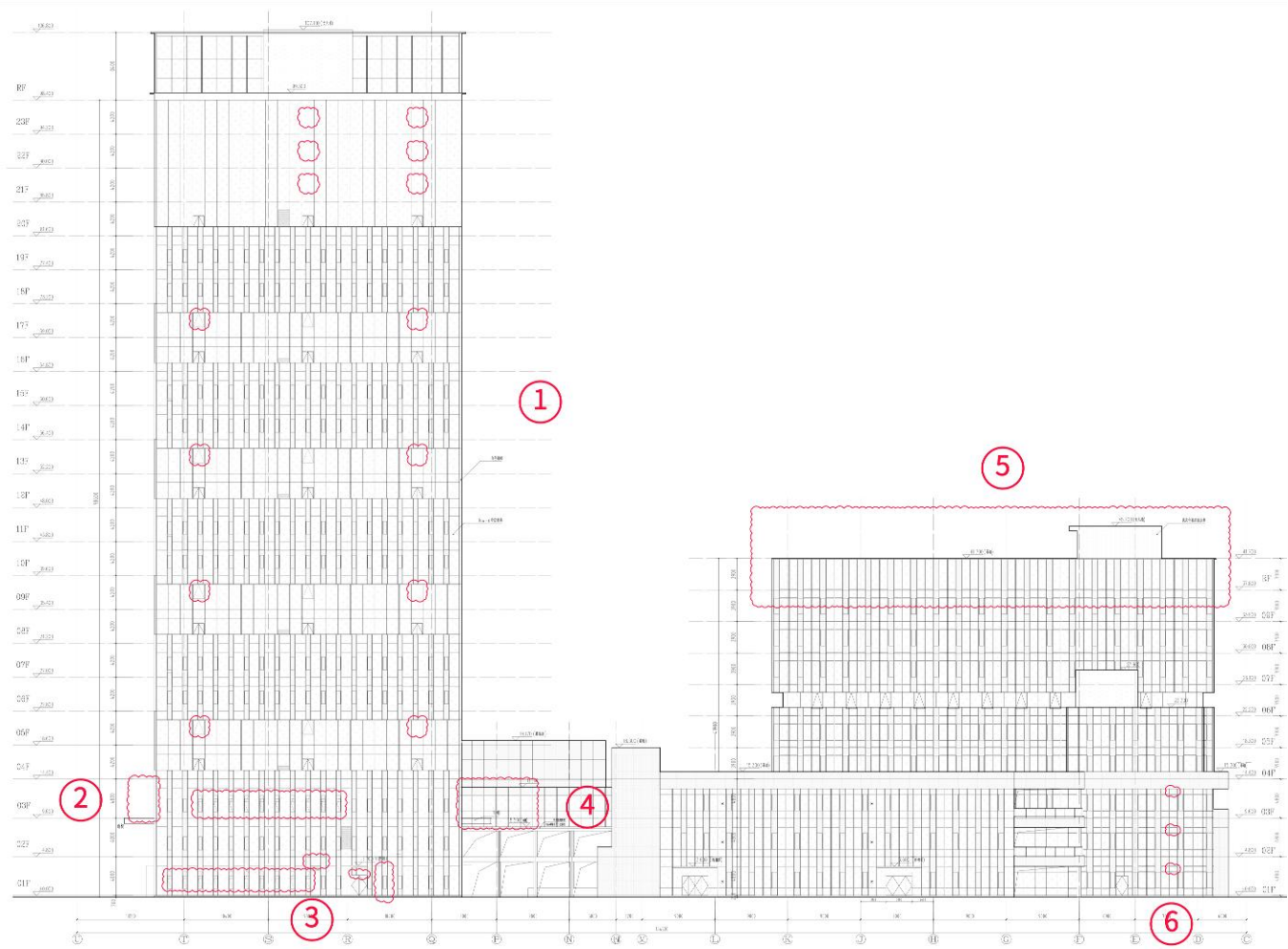
西立面图变更后
