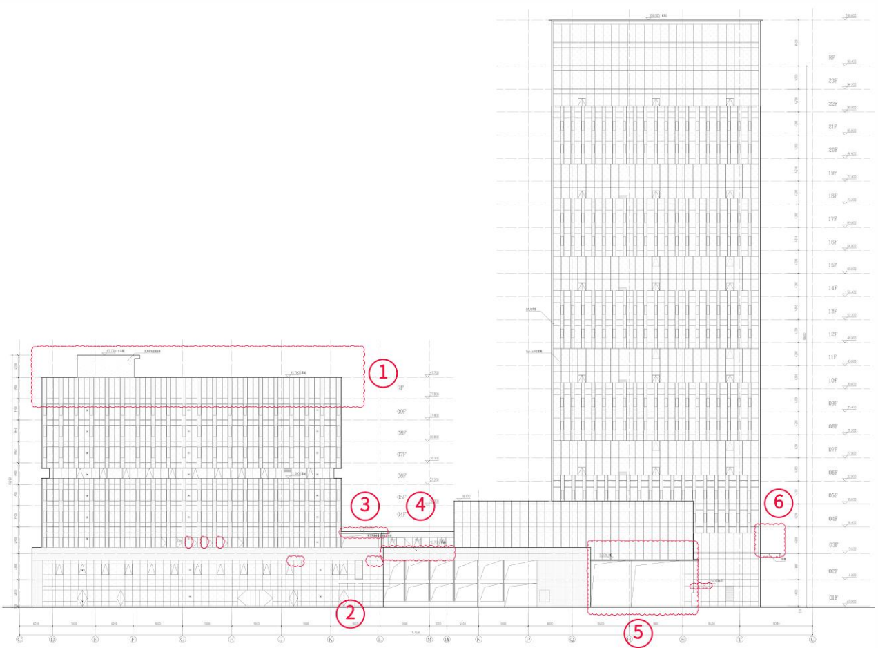
东立面图变更后
