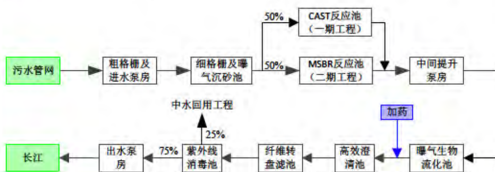
图 4-2 珠江污水处理厂工艺流程图
